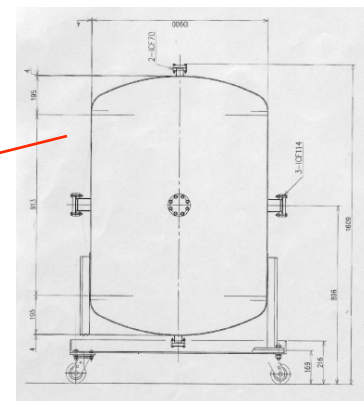
0.75m 3 バッファタンク (製作中)
