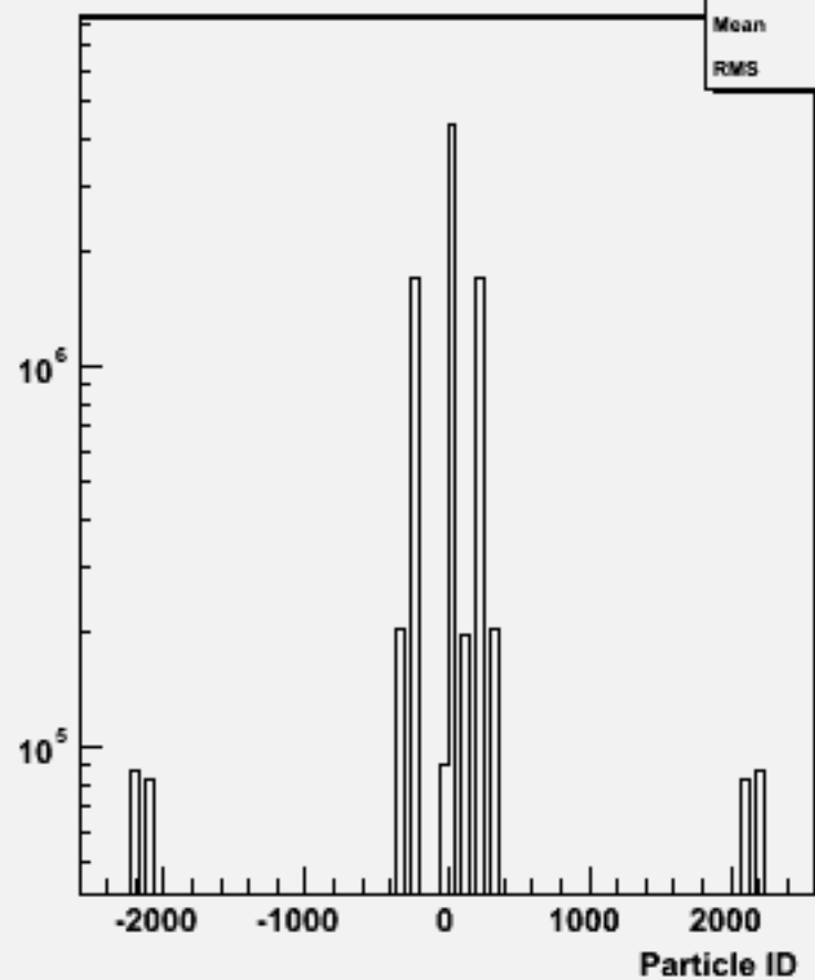
Particle ID : p106023 physsim-ttz-6q_zqq
