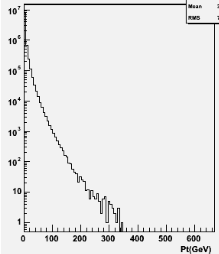
Particle Pt : p106023 physsim-ttz-6q_zqq
