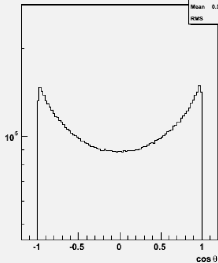
Particle cos \theta : p106023 physsim-ttz-6q_zqq
