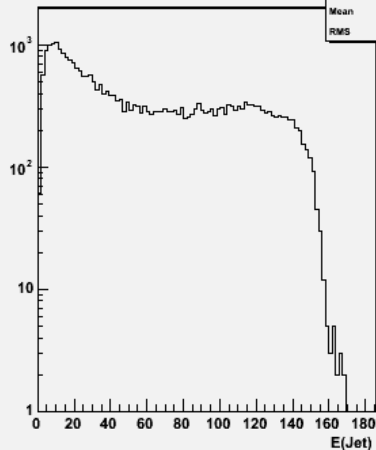
Jet energies(All jets)w104056 aa_n2n2uu_o
