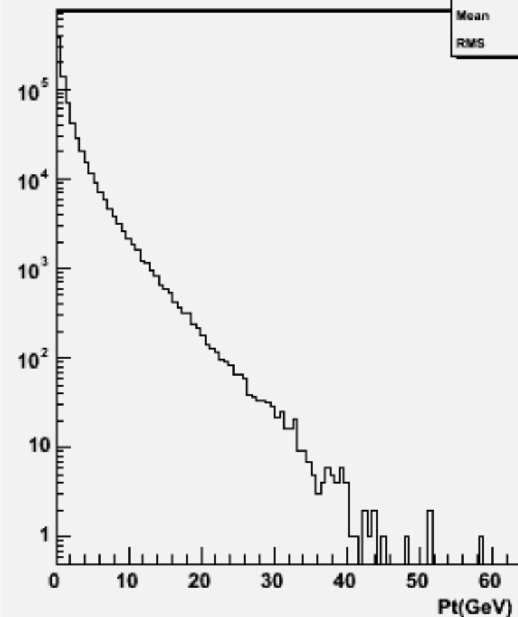
Particle Pt : w104046 aa_cssc_o
