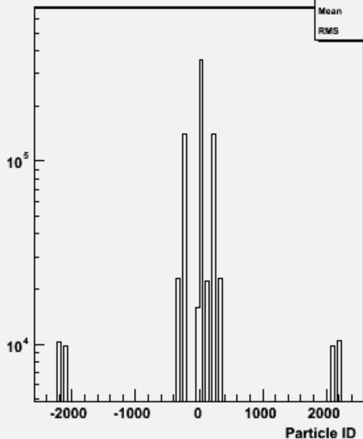
Particle ID : w104046 aa_cssc_o
