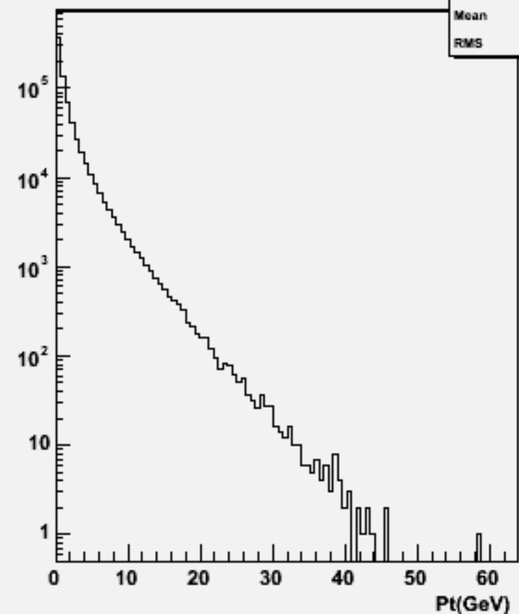
Particle Pt : w104045 aa_cssc_o
