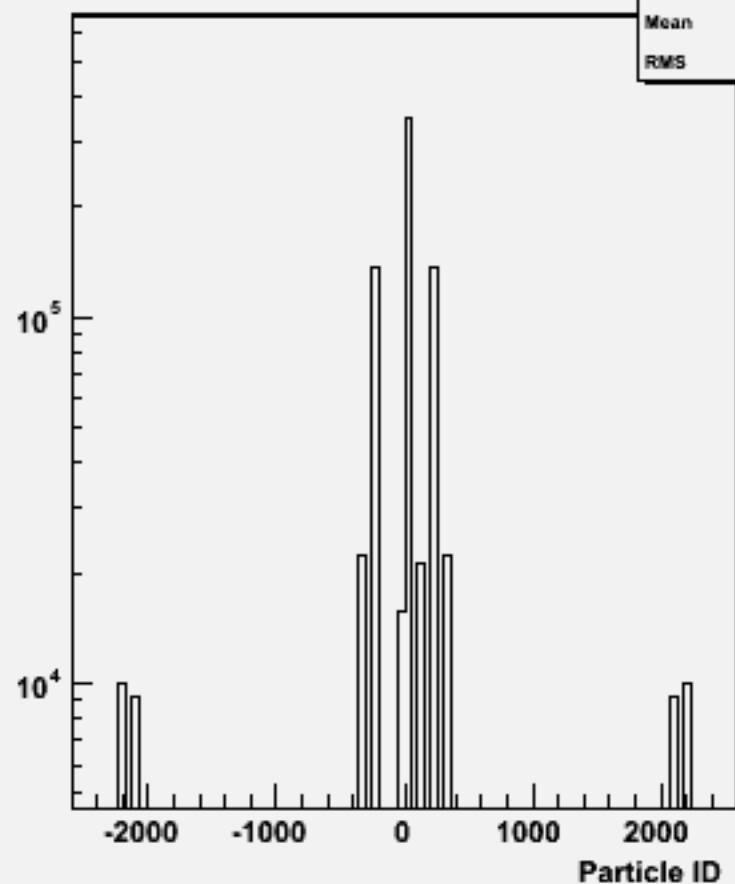
Particle ID : w104045 aa_cssc_o
