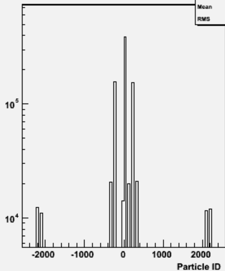
Particle ID : w104040 aa_csdu_o
