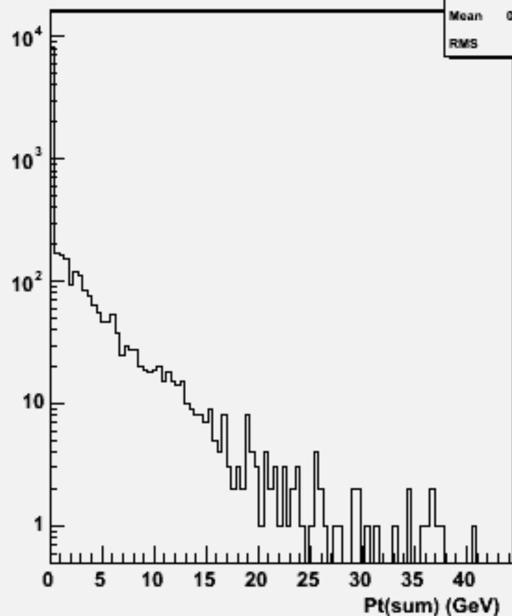
Pt Sum: w104040 aa_csdu_o
