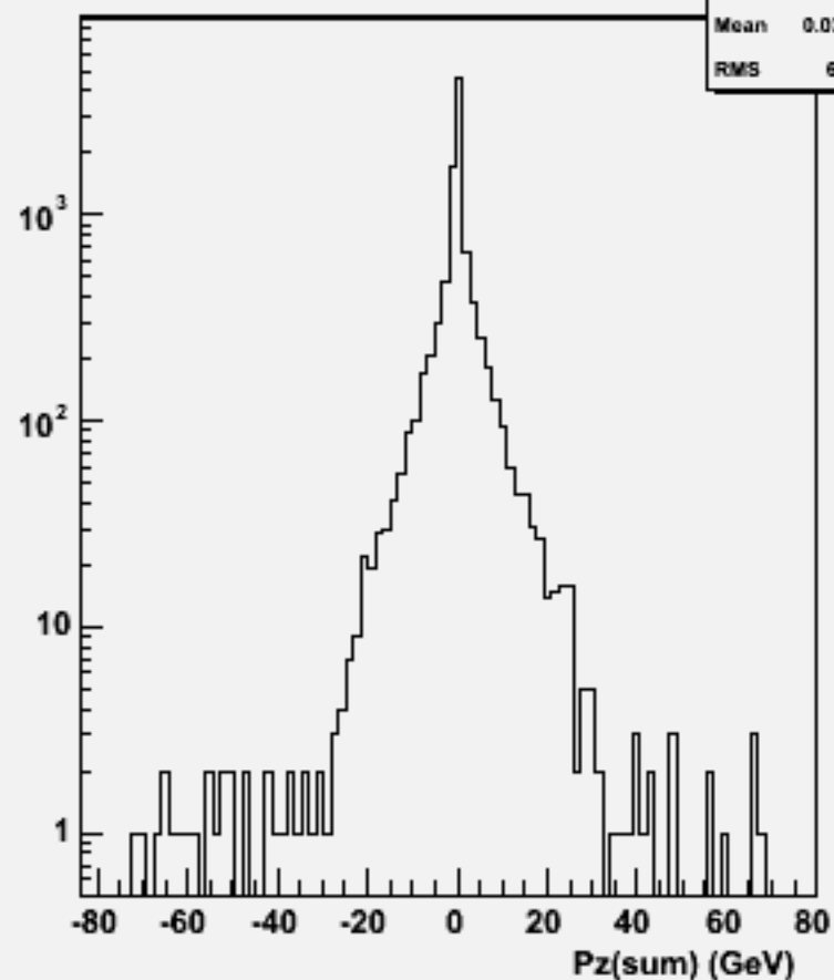
Pz Sum: w104040 aa_csdu_o
