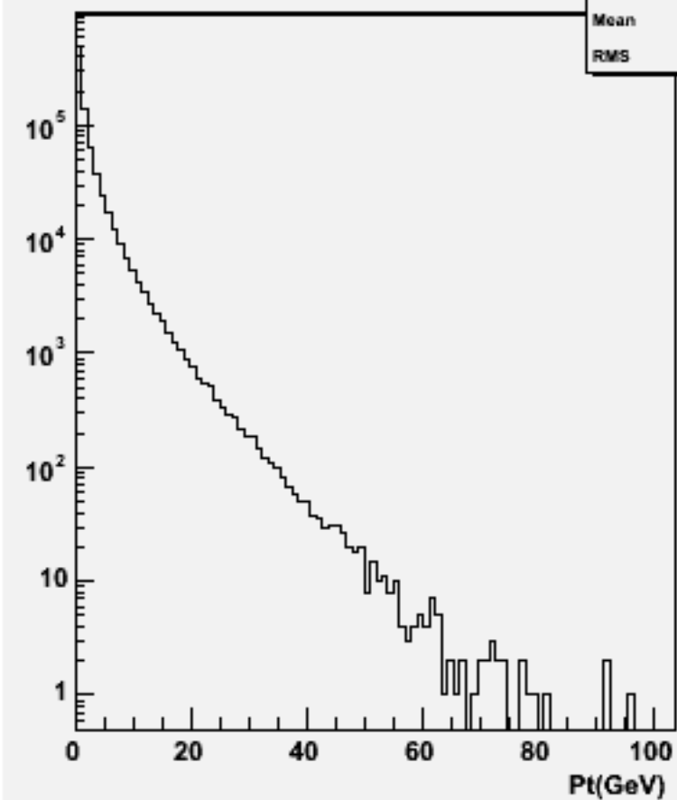
Particle Pt : w104040 aa_csdu_o
