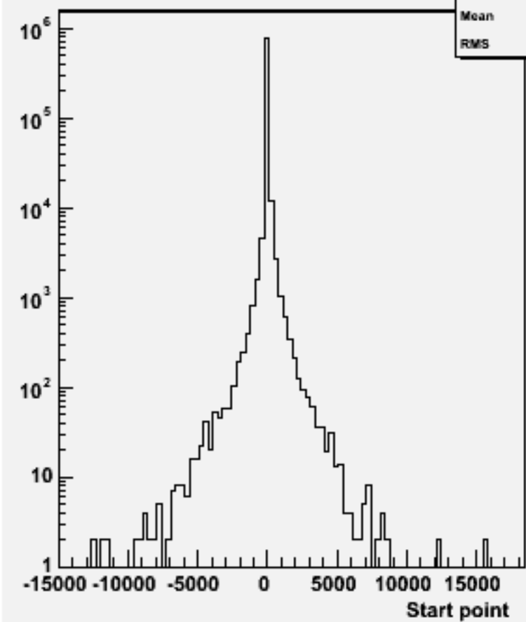
Start point Z : w104040 aa_csdu_o
