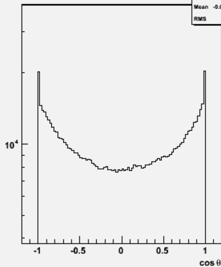
Particle \cos\theta : w104040 aa_csdu_o
