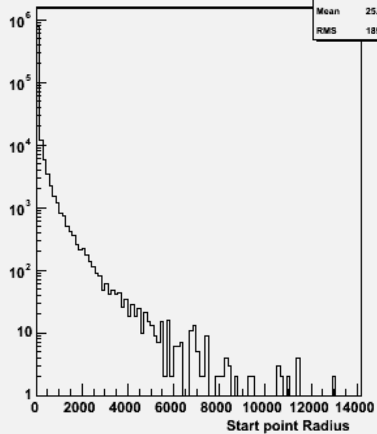
Start point R : w104040 aa_csdu_o
