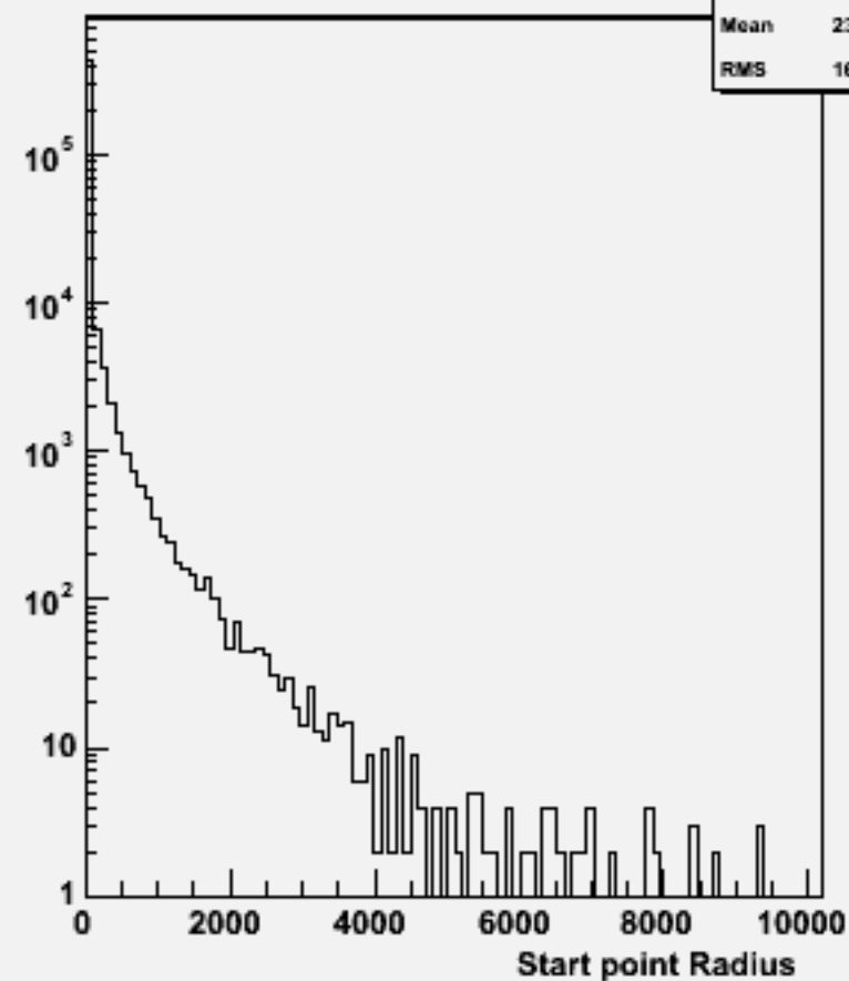
Start point R : w104038 aa_cse3n3_o
