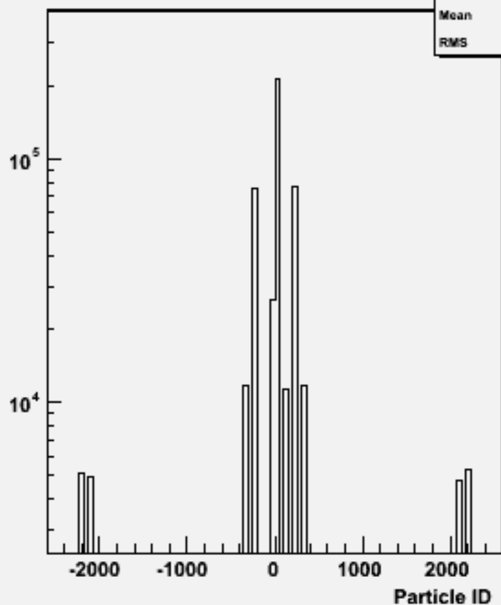
Particle ID : w104038 aa_cse3n3_o
