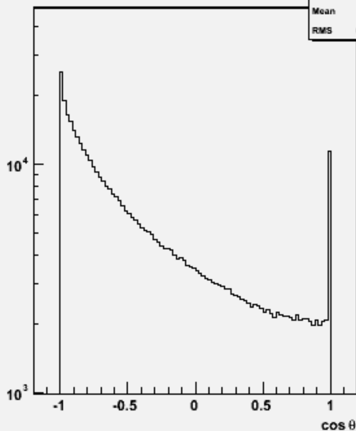
Particle cos \theta : w104038 aa_cse3n3_o
