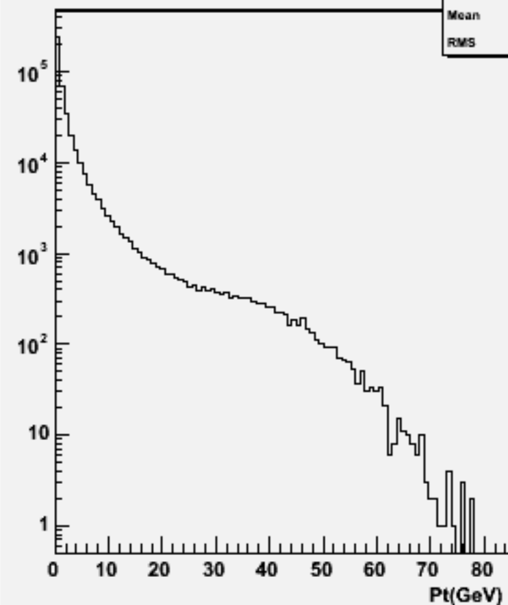
Particle Pt : w104038 aa_cse3n3_o
