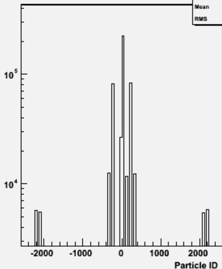
Particle ID : w104036 aa_cse3n3_o
