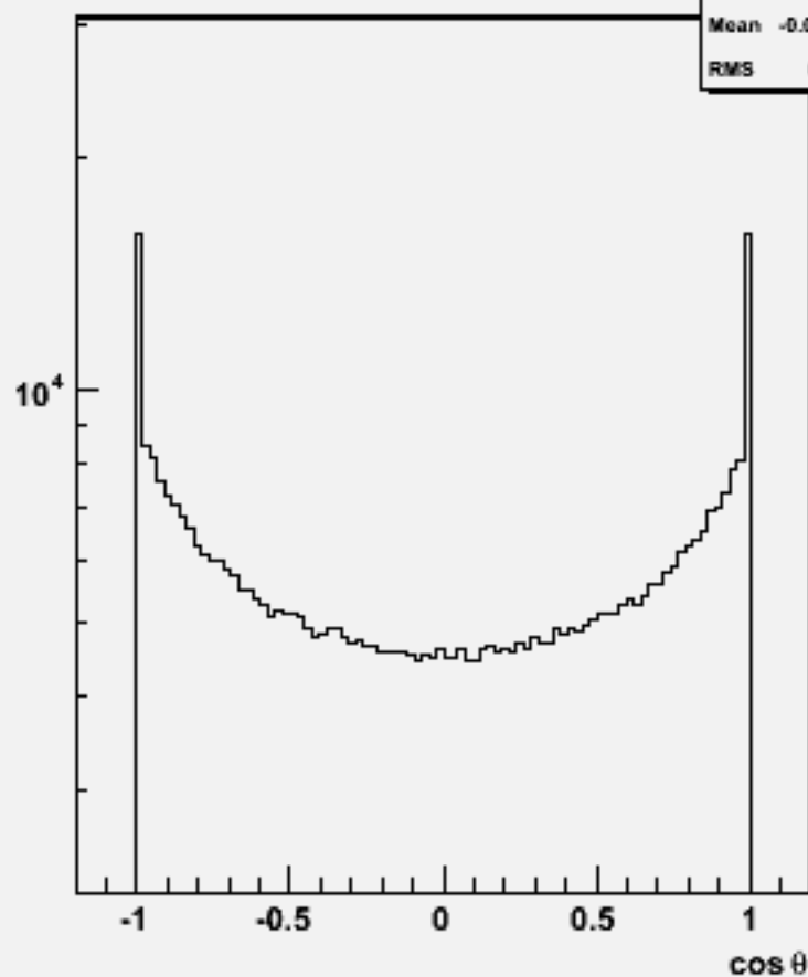
Particle cos \theta : w104036 aa_cse3n3_o
