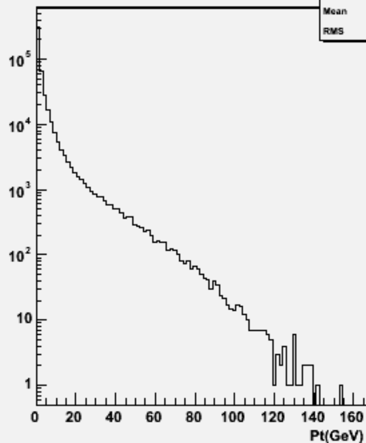
Particle Pt : w104036 aa_cse3n3_o
