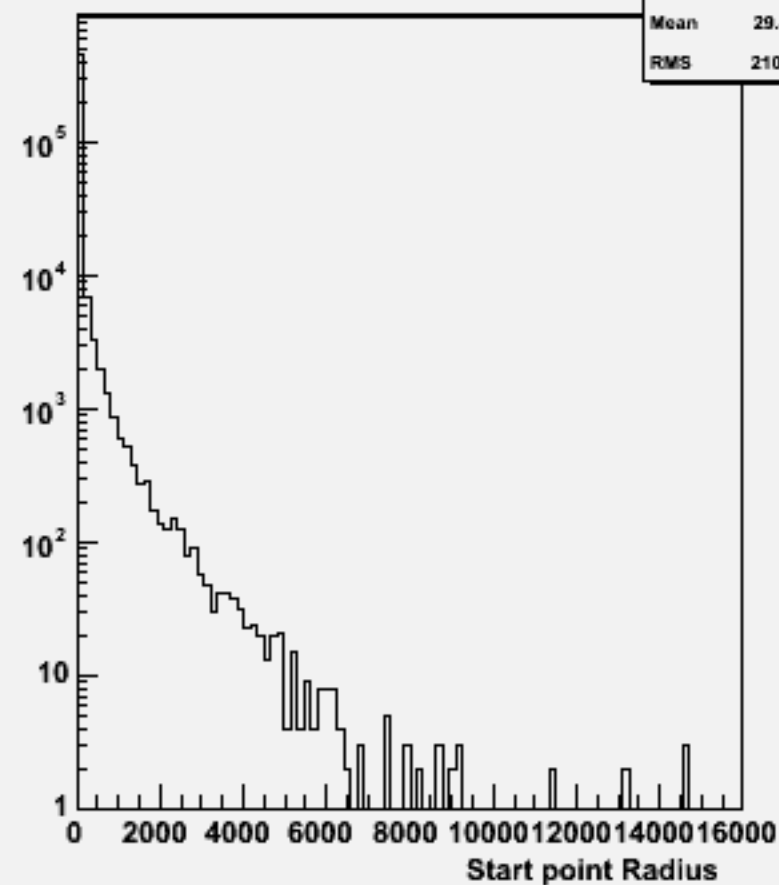
Start point R : w104036 aa_cse3n3_o
