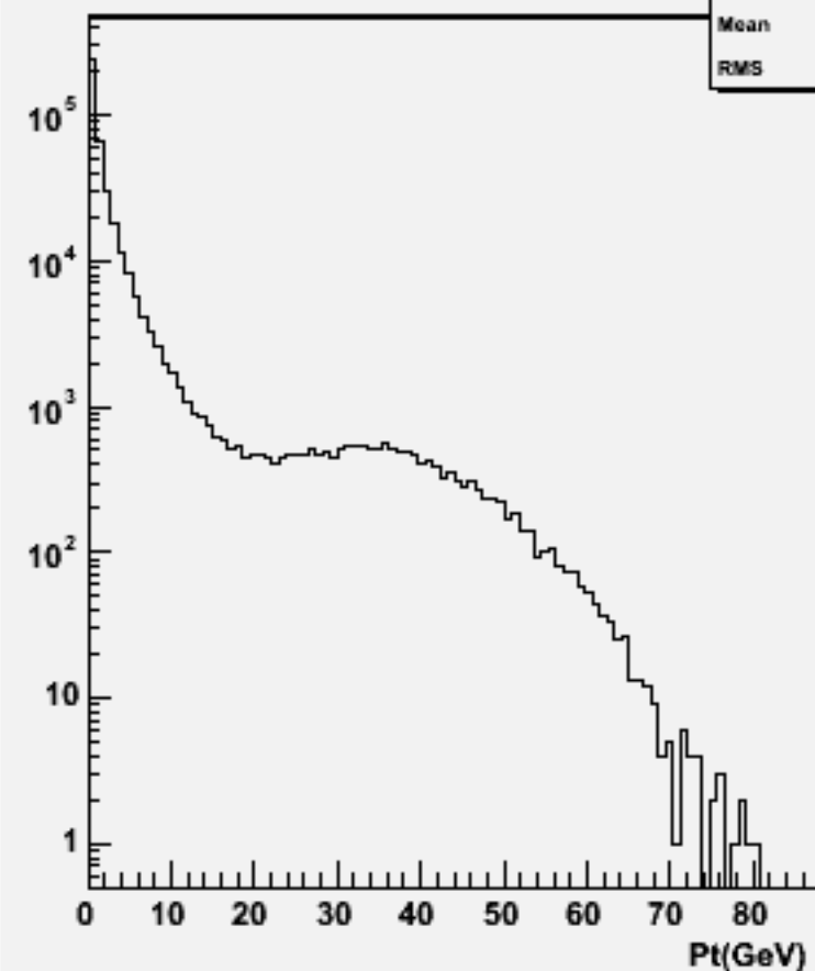
Particle Pt : w104034 aa_cse2n2_o
