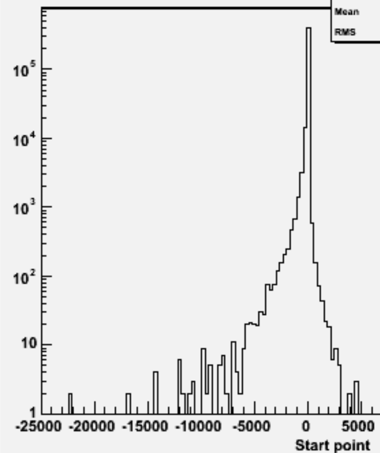
Start point Z : w104034 aa_cse2n2_o
