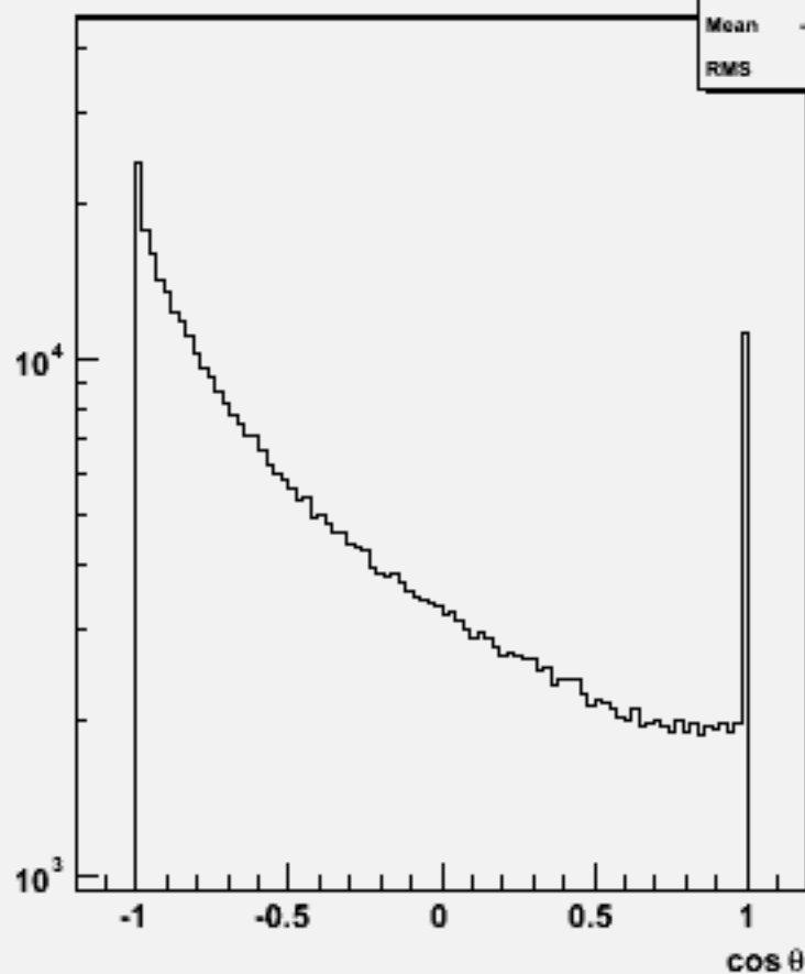
Particle cos \theta : w104034 aa_cse2n2_o
