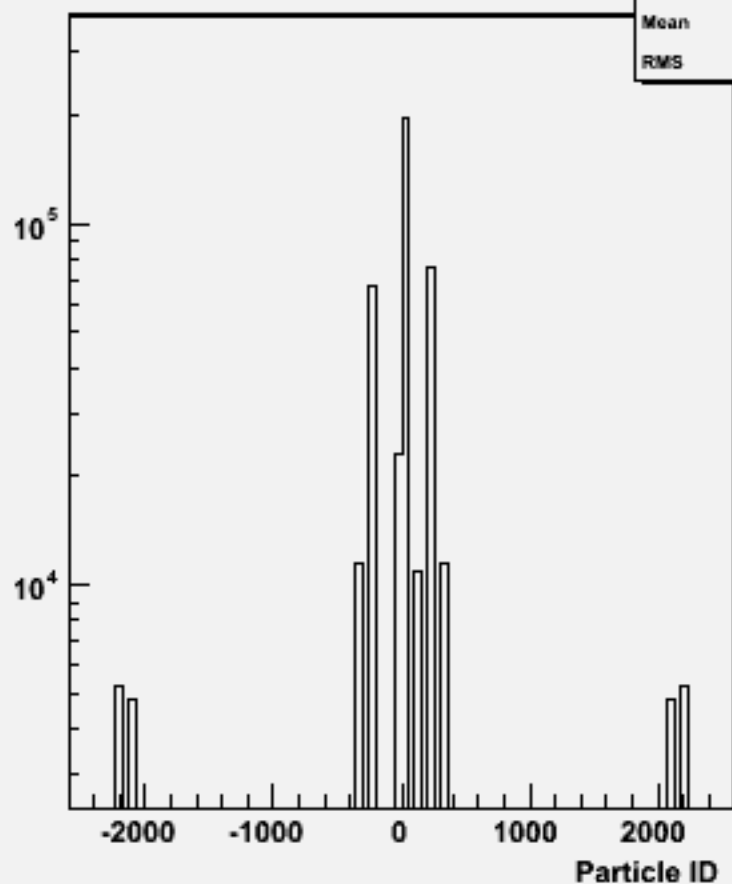
Particle ID : w104034 aa_cse2n2_o
