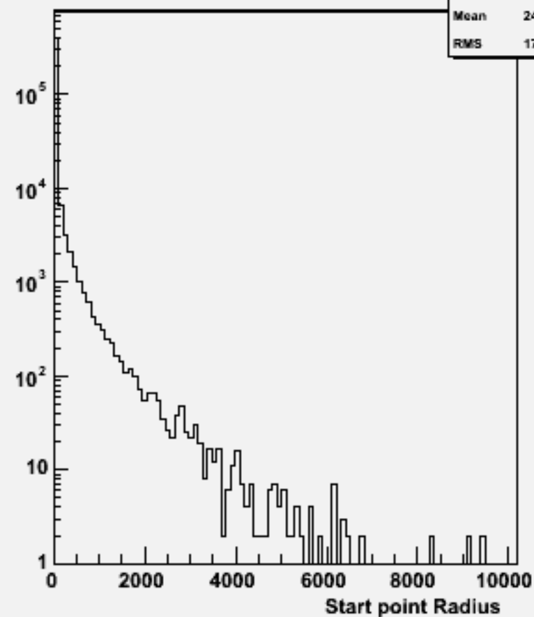
Start point R : w104034 aa_cse2n2_o
