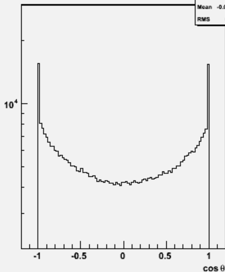
Particle cos \theta : w104032 aa_cse2n2_o
