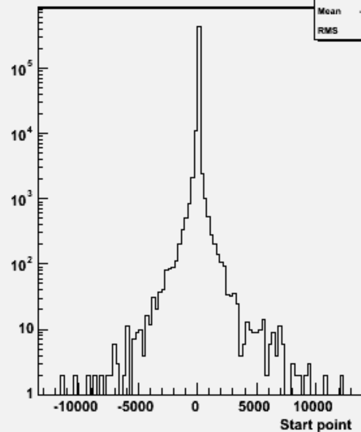
Start point Z : w104032 aa_cse2n2_o
