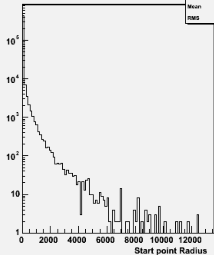
Start point R : w104032 aa_cse2n2_o
