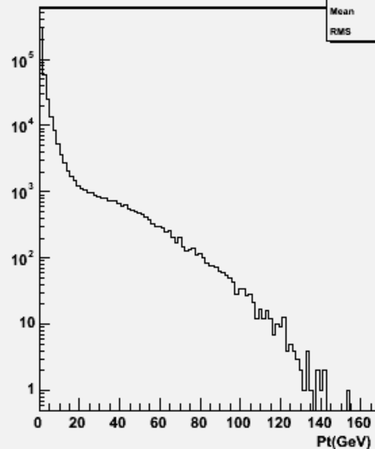
Particle Pt : w104032 aa_cse2n2_o
