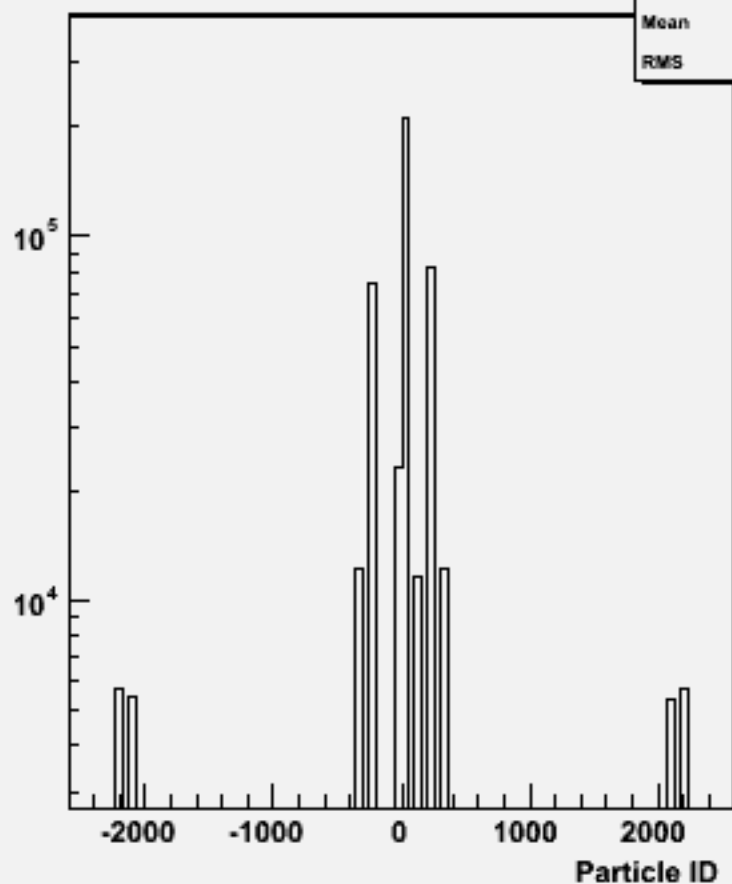
Particle ID : w104032 aa_cse2n2_o
