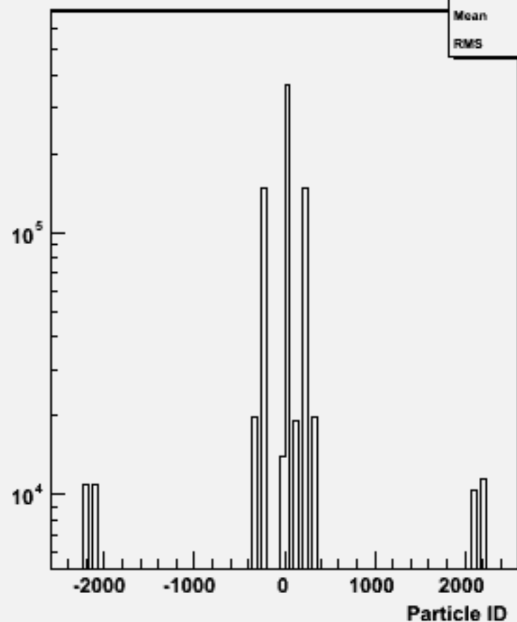
Particle ID : w104026 aa_udsc_o
