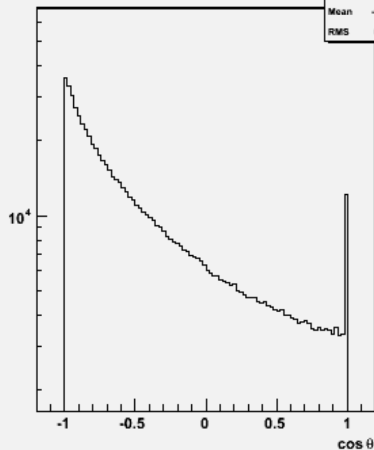
Particle cosθ : w104026 aa_udsc_o
