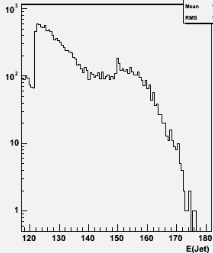
Jet energies(All jets)w104026 aa_udsc_o
