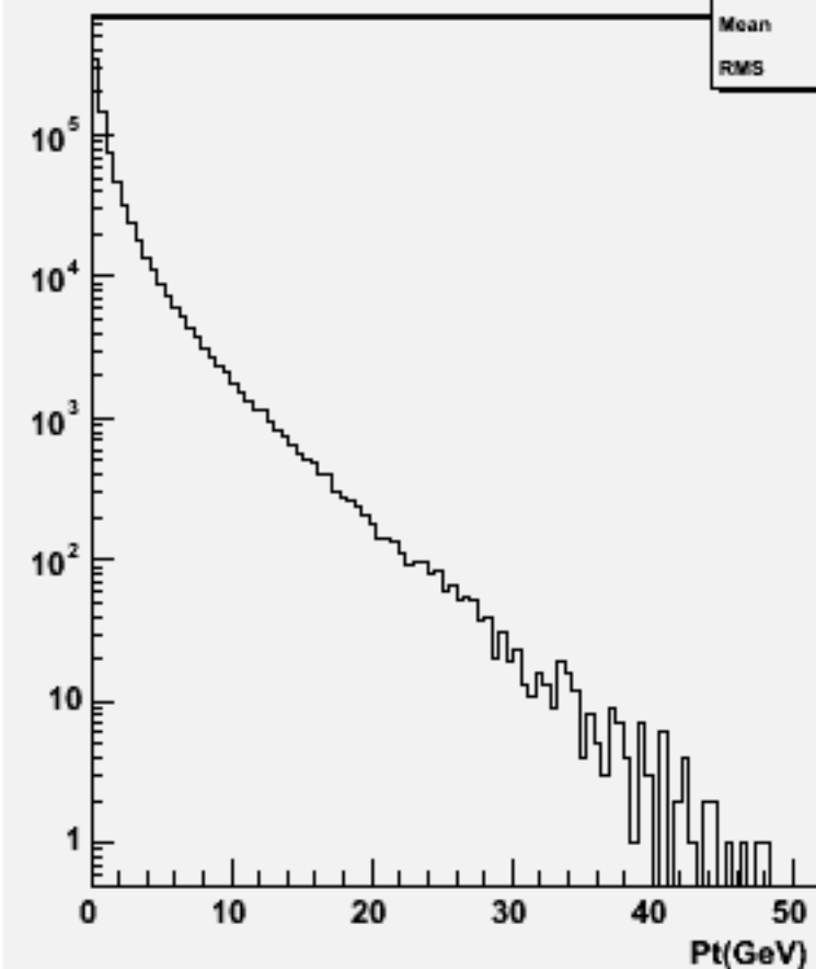
Particle Pt : w104026 aa_udsc_o
