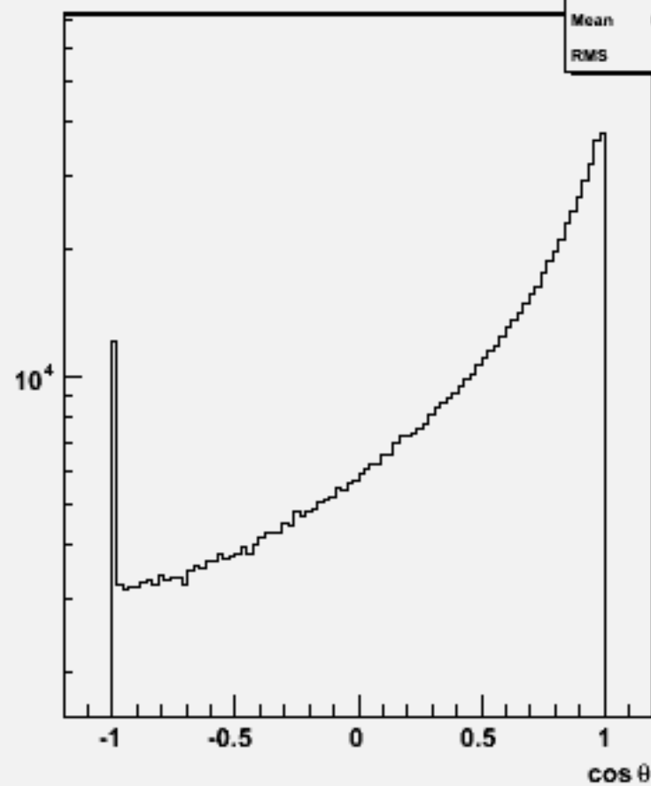
Particle cosθ : w104025 aa_udsc_o
