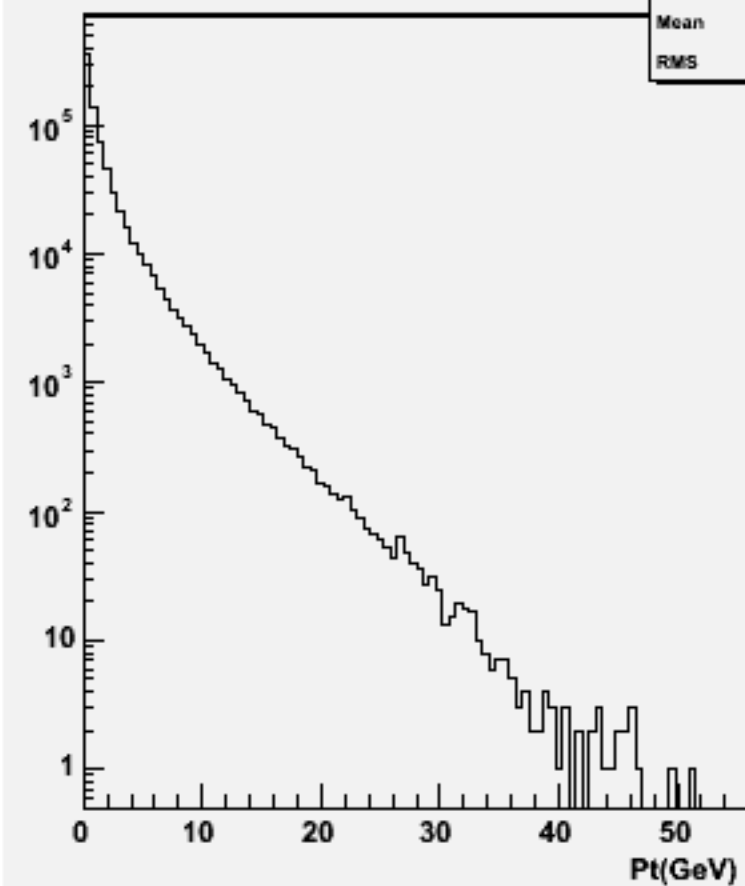
Particle Pt : w104025 aa_udsc_o
