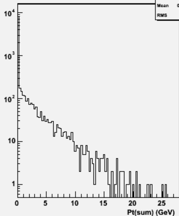
Pt Sum: w104025 aa_udsc_o
