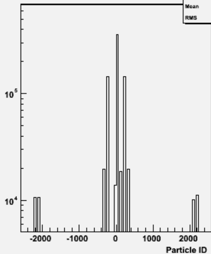
Particle ID : w104025 aa_udsc_o
