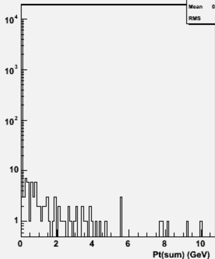
Pt Sum: w104022 aa_uddu_o
