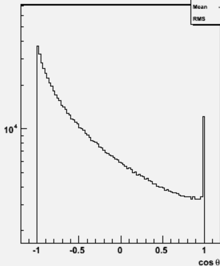
Particle \cos\theta : w104022 aa_uddu_o
