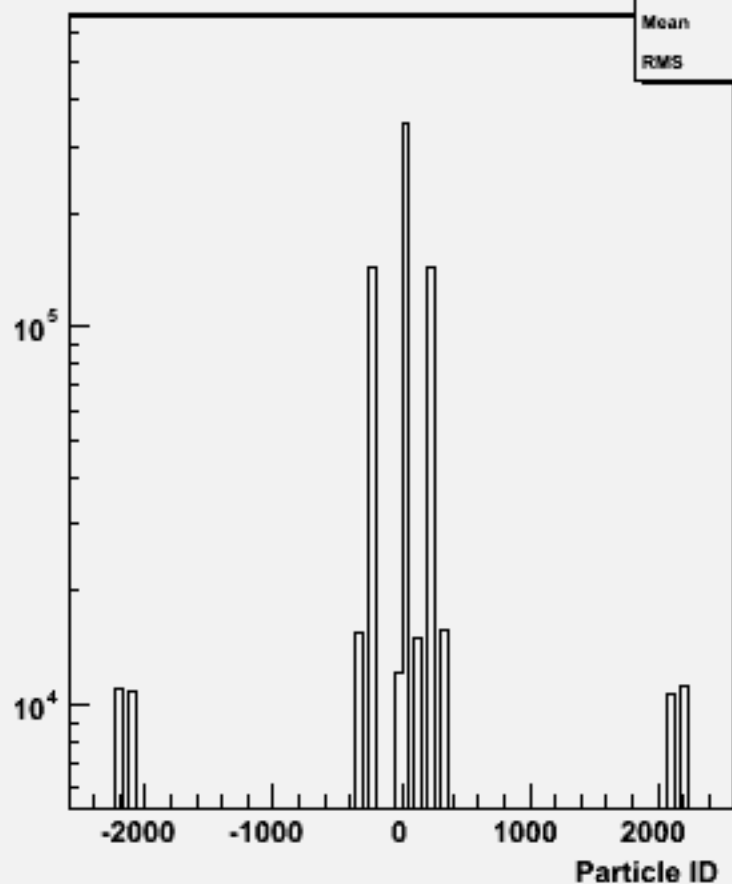
Particle ID : w104022 aa_uddu_o
