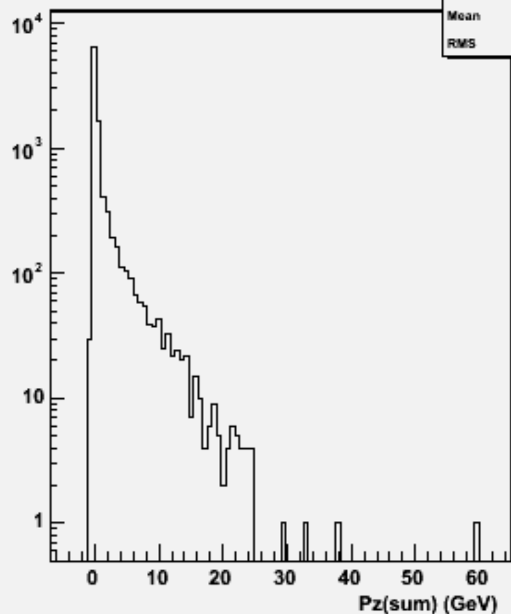
Pz Sum: w104022 aa_uddu_o
