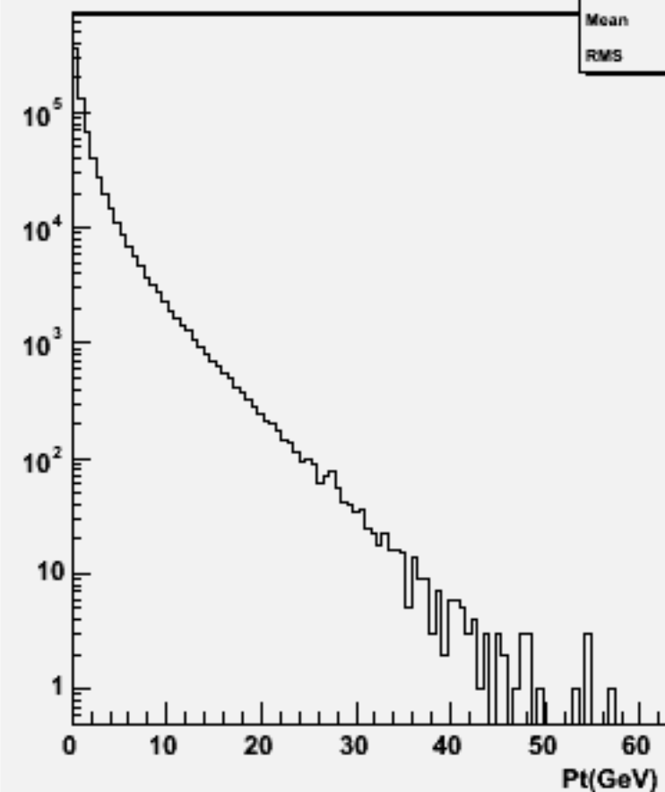
Particle Pt : w104022 aa_uddu_o
