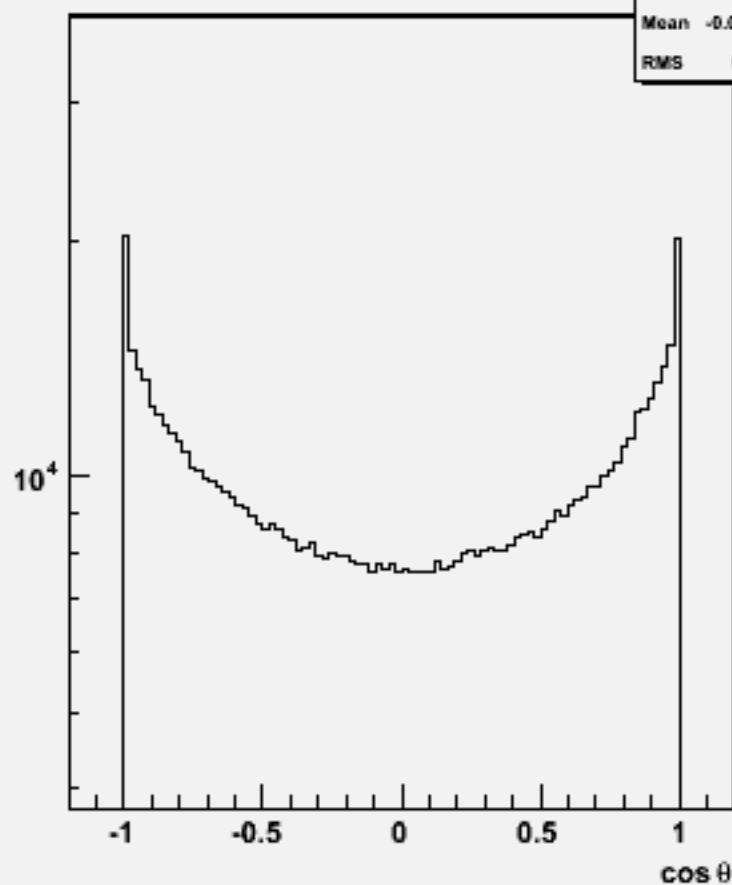
Particle \cos\theta : w104020 aa_uddu_o
