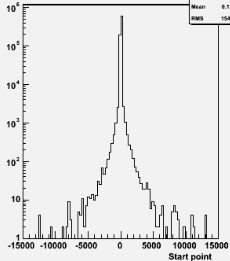
Start point Z : w104020 aa_uddu_o
