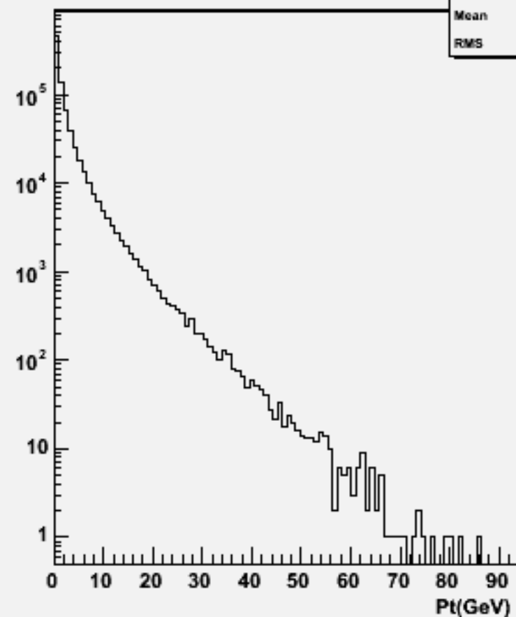
Particle Pt : w104020 aa_uddu_o
