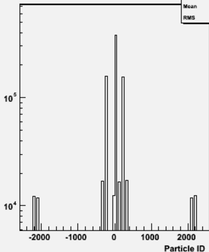
Particle ID : w104020 aa_uddu_o
