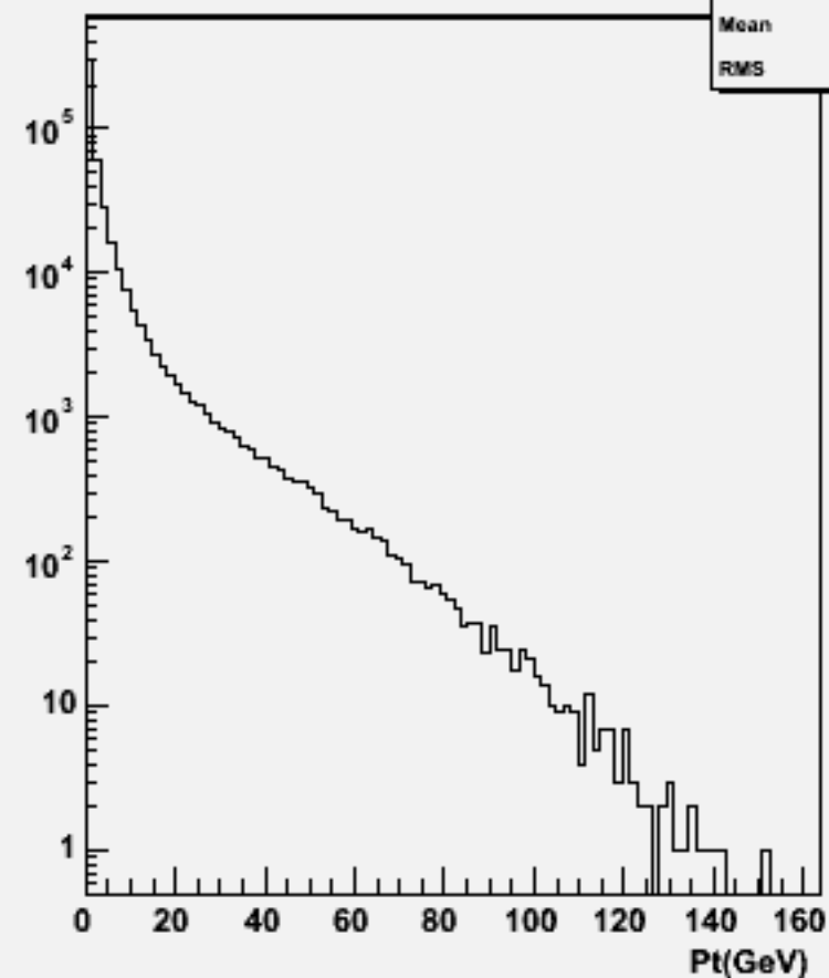
Particle Pt : w104016 aa_ude3n3_o
