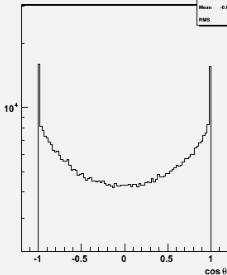
Particle cos \theta : w104016 aa_ude3n3_o
