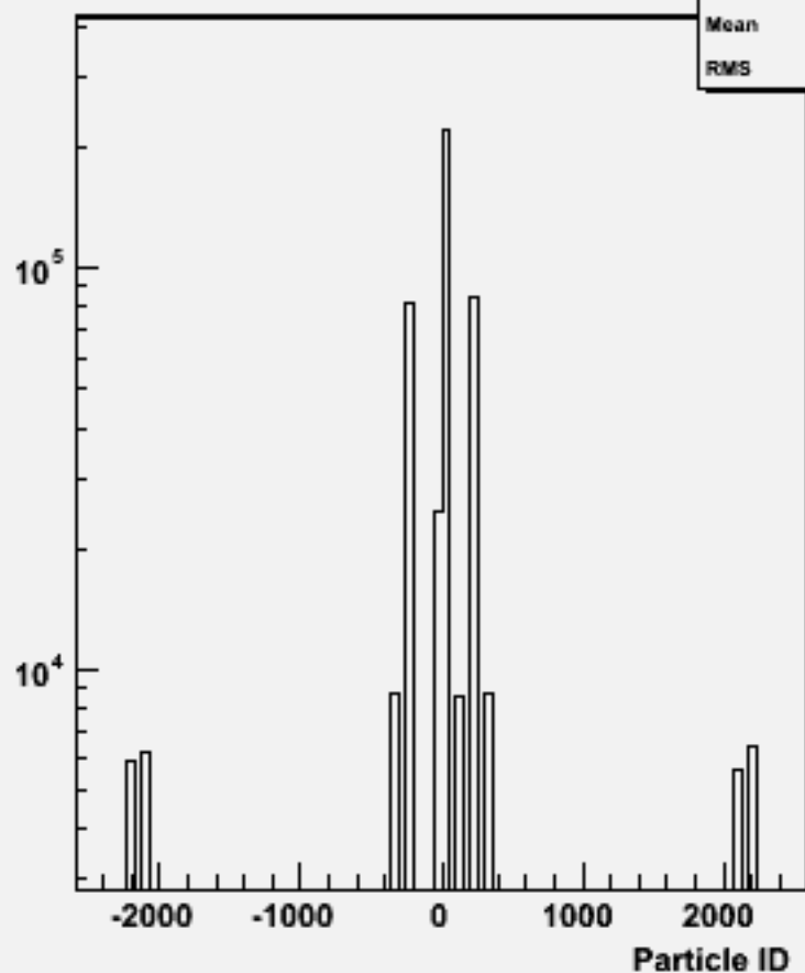
Particle ID : w104016 aa_ude3n3_o
