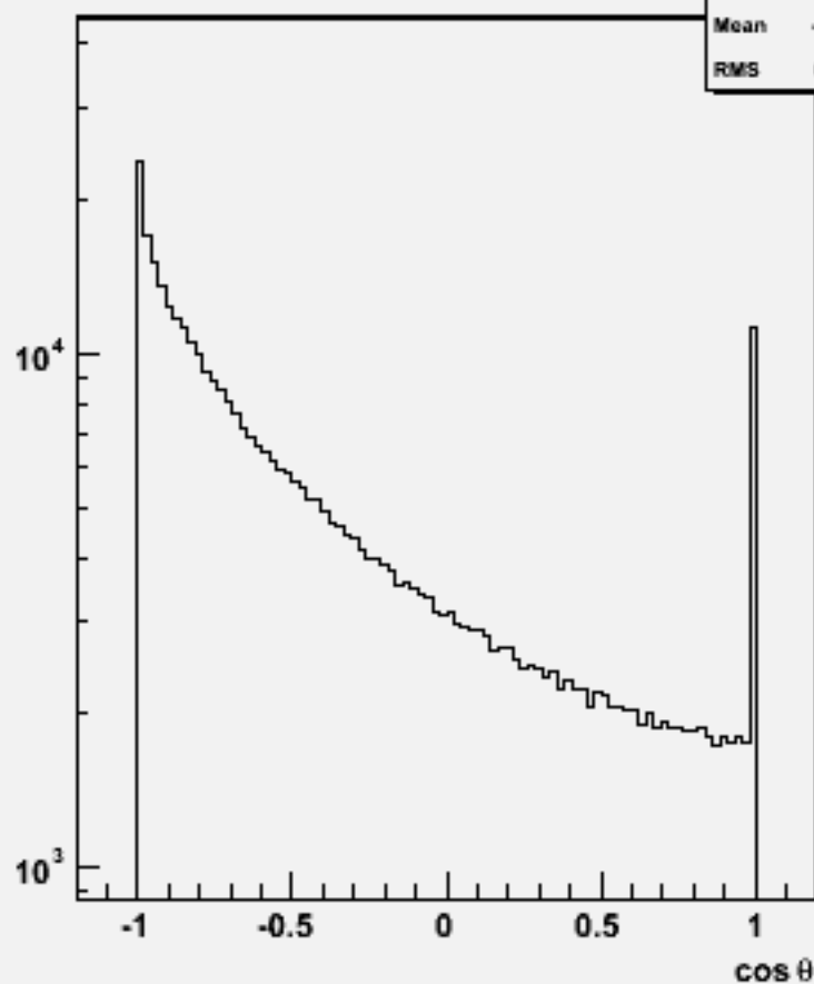
Particle cos \theta : w104014 aa_ude2n2_o
