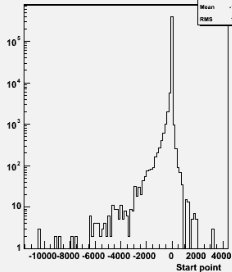
Start point Z : w104014 aa_ude2n2_o
