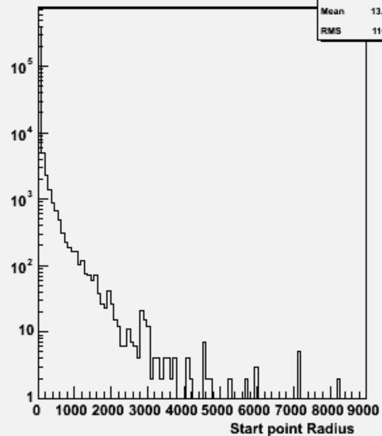
Start point R : w104014 aa_ude2n2_o
