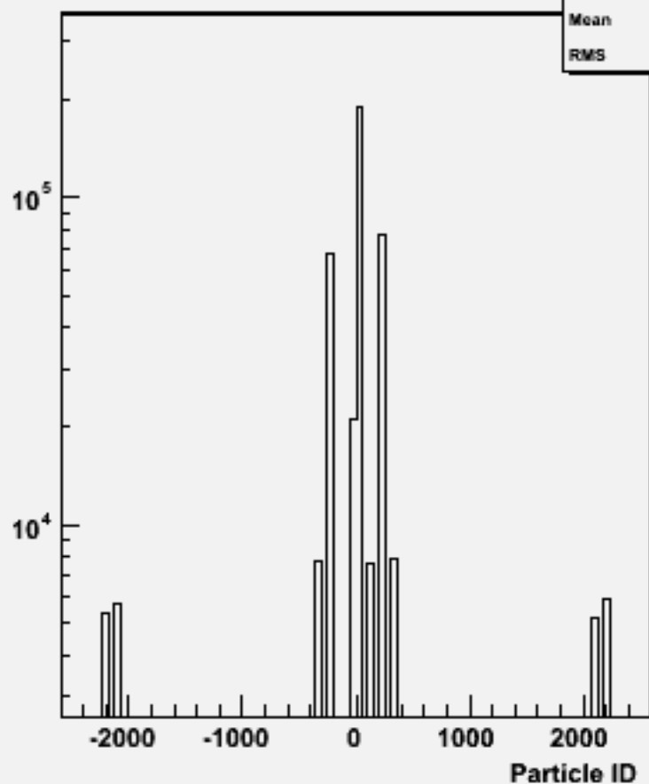
Particle ID : w104014 aa_ude2n2_o
