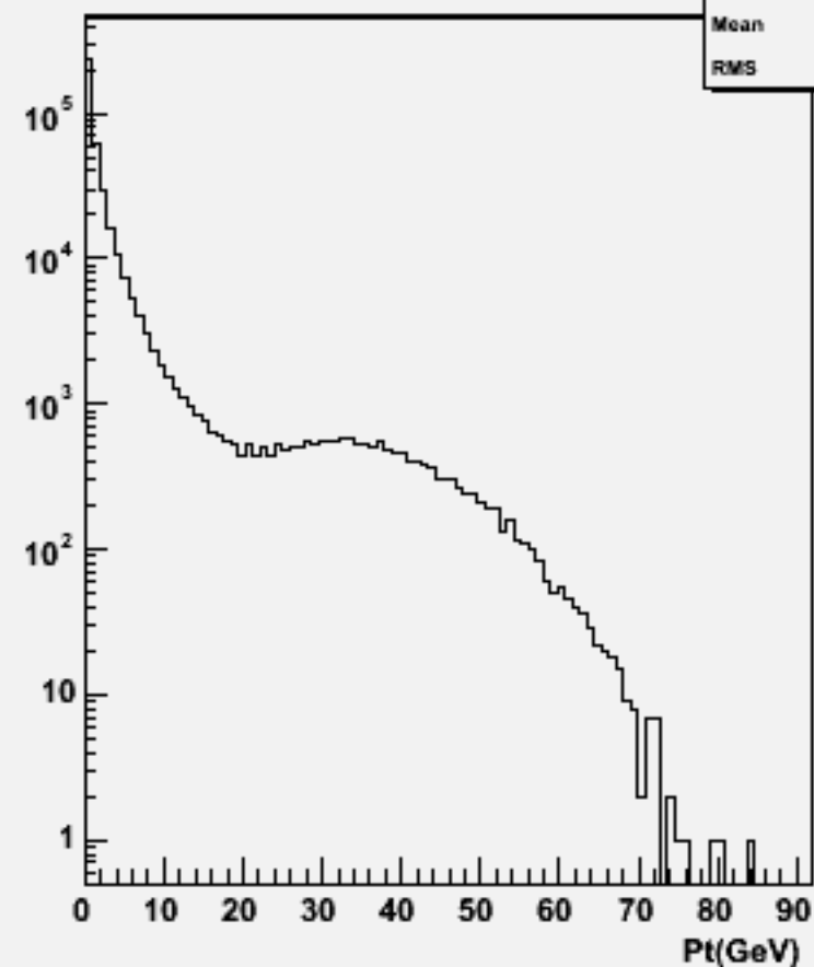
Particle Pt : w104014 aa_ude2n2_o
