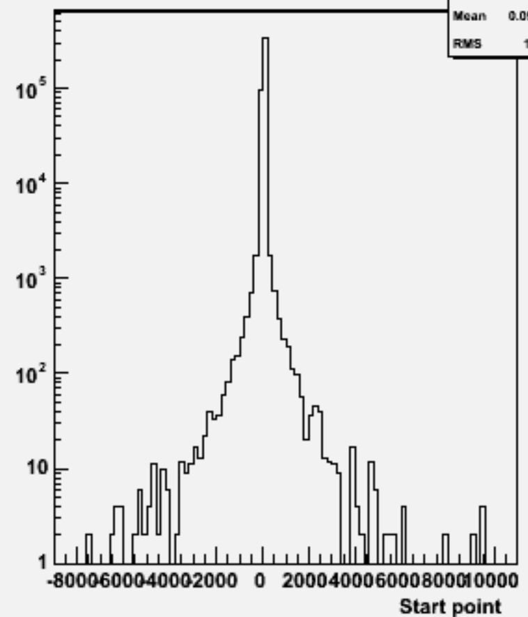
Start point Z : w104012 aa_ude2n2_o
