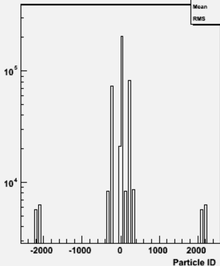
Particle ID : w104012 aa_ude2n2_o
