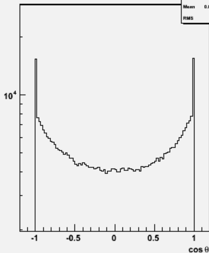
Particle cos \theta : w104012 aa_ude2n2_o
