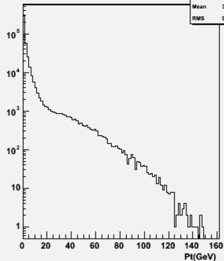
Particle Pt : w104012 aa_ude2n2_o
