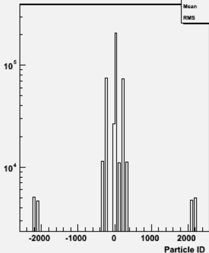
Particle ID : w104005 aa_n3e3sc_o
