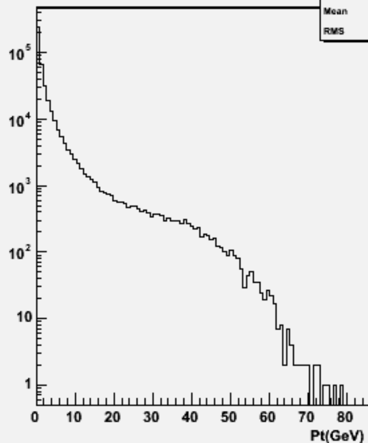
Particle Pt : w104005 aa_n3e3sc_o
