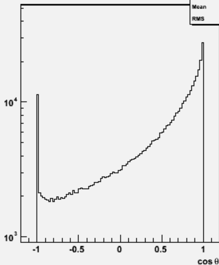
Particle cos \theta : w104005 aa_n3e3sc_o
