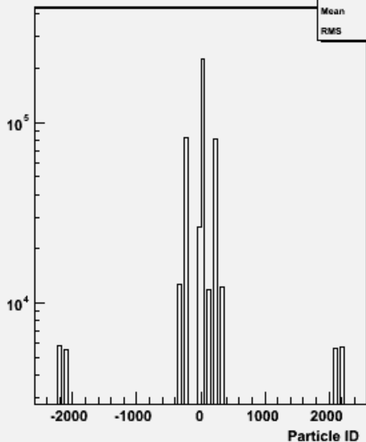
Particle ID : w104004 aa_n3e3sc_o
