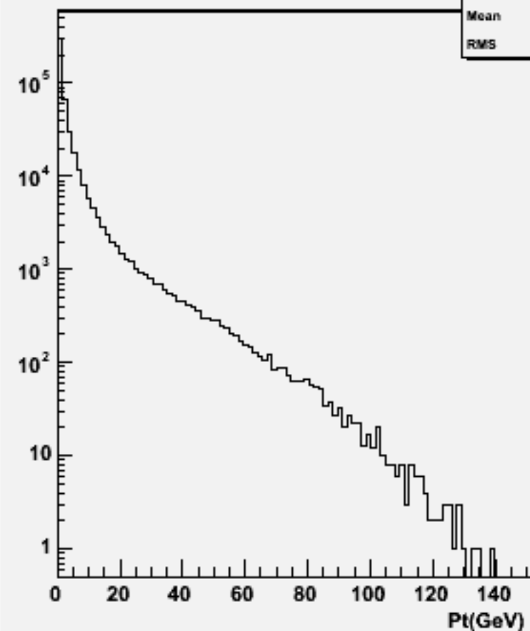
Particle Pt : w104004 aa_n3e3sc_o
