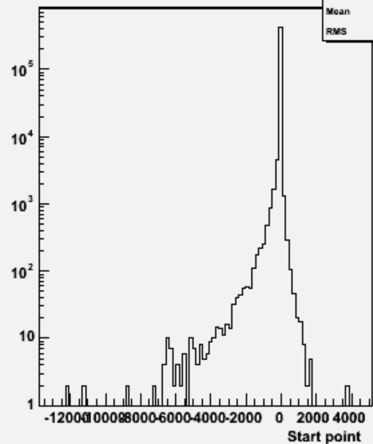
Start point Z : w104002 aa_n3e3du_o
