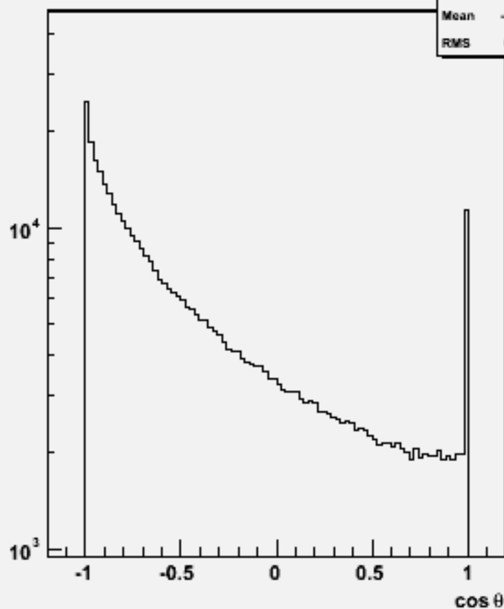
Particle cos \theta : w104002 aa_n3e3du_o
