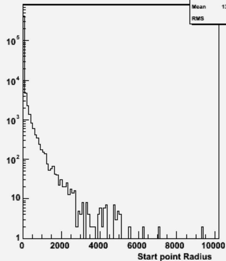
Start point R : w104002 aa_n3e3du_o
