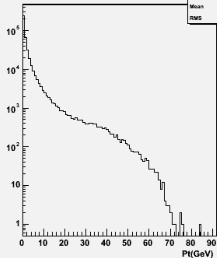
Particle Pt : w104002 aa_n3e3du_o
