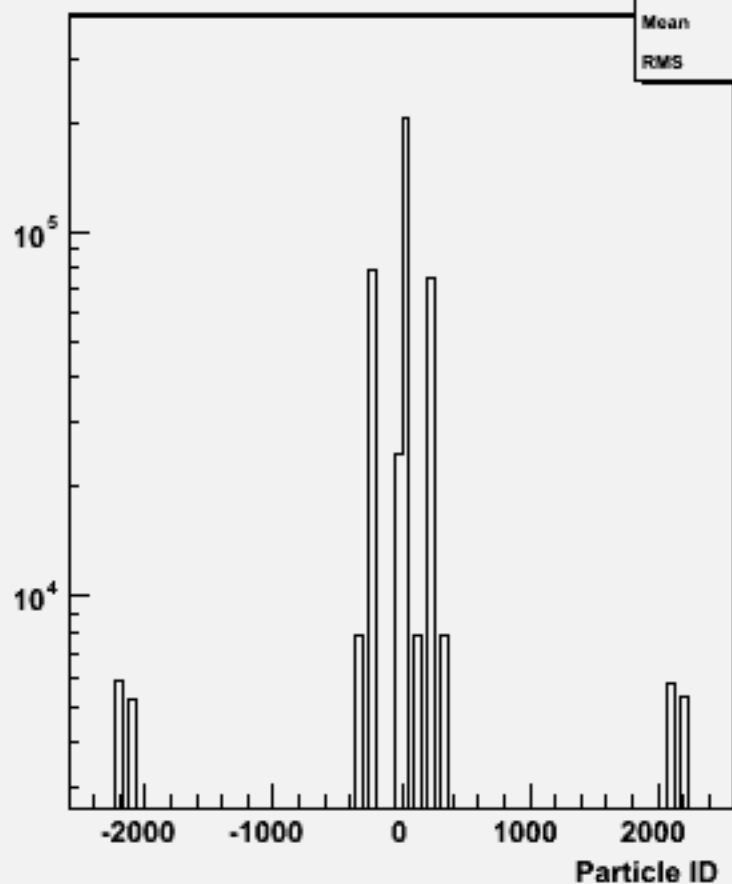
Particle ID : w104002 aa_n3e3du_o
