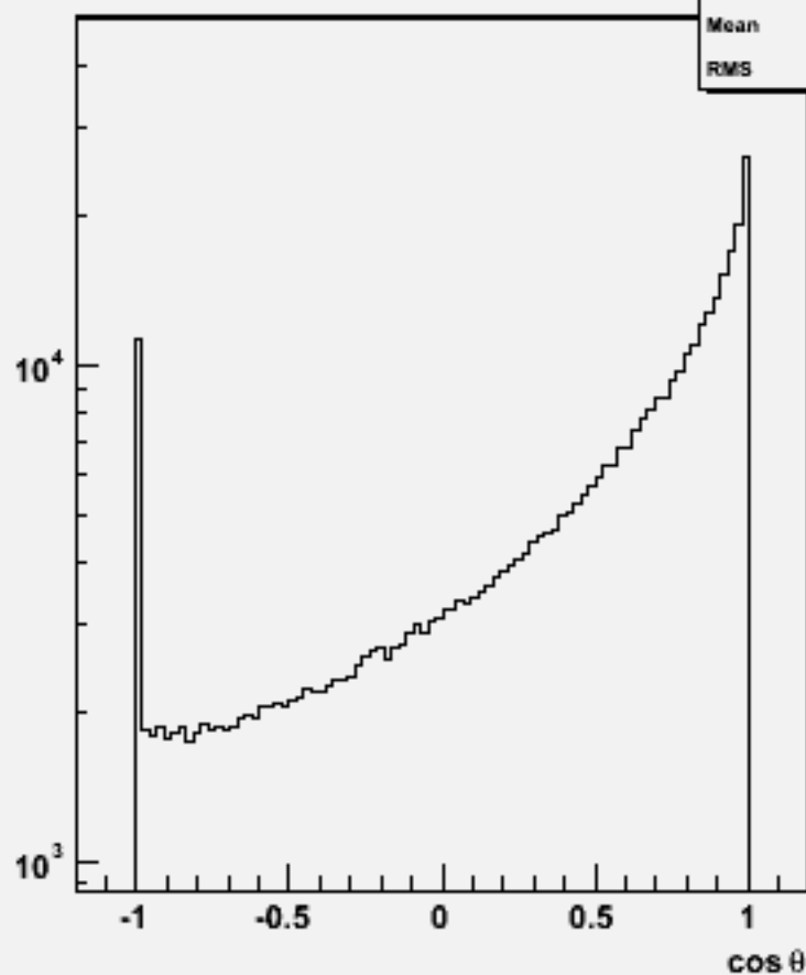
Particle cos \theta : w104001 aa_n3e3du_o
