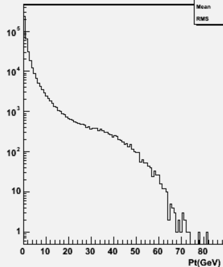
Particle Pt : w104001 aa_n3e3du_o
