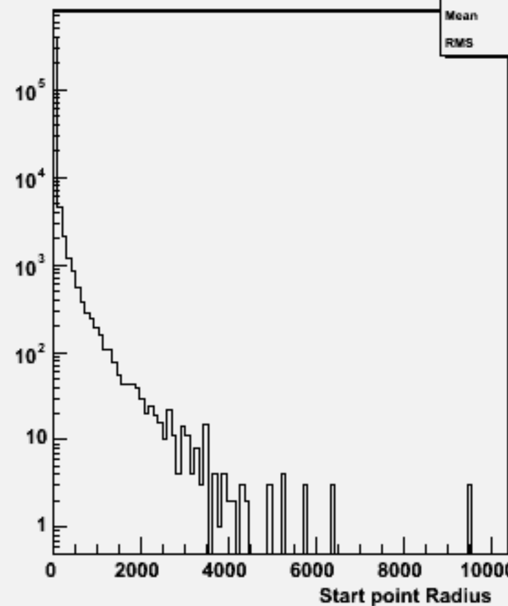
Start point R : w104001 aa_n3e3du_o
