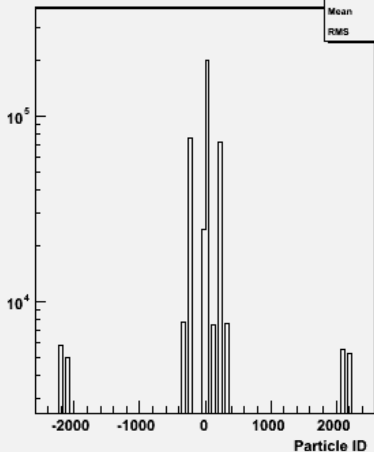
Particle ID : w104001 aa_n3e3du_o
