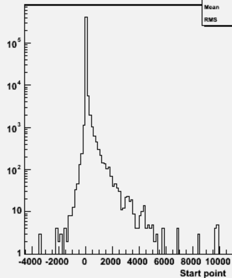
Start point Z : w104001 aa_n3e3du_o
