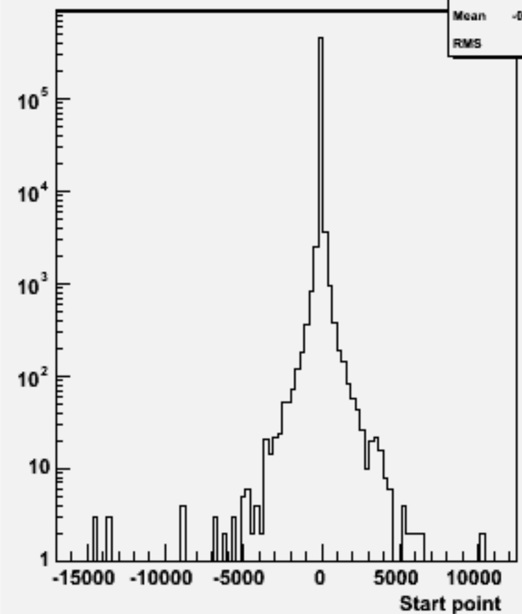
Start point Z : w104000 aa_n3e3du_o
