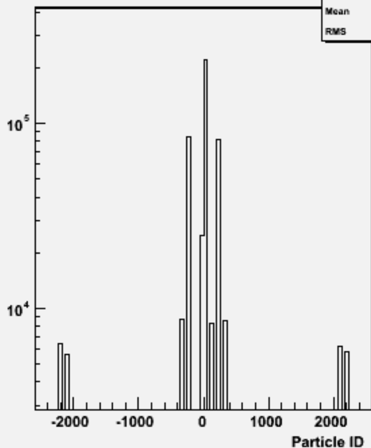
Particle ID : w104000 aa_n3e3du_o
