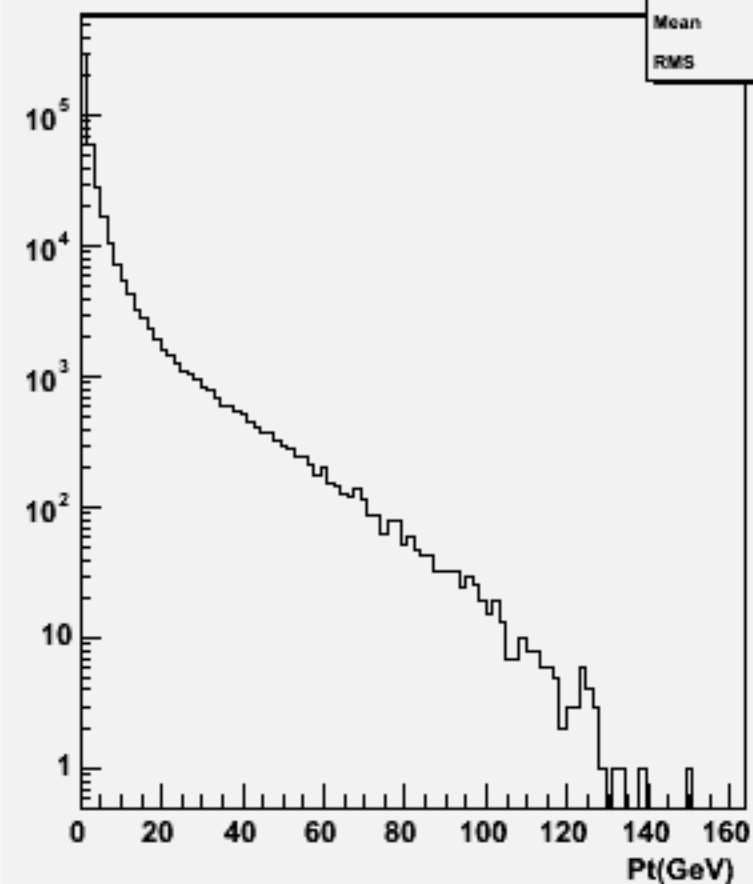
Particle Pt : w104000 aa_n3e3du_o
