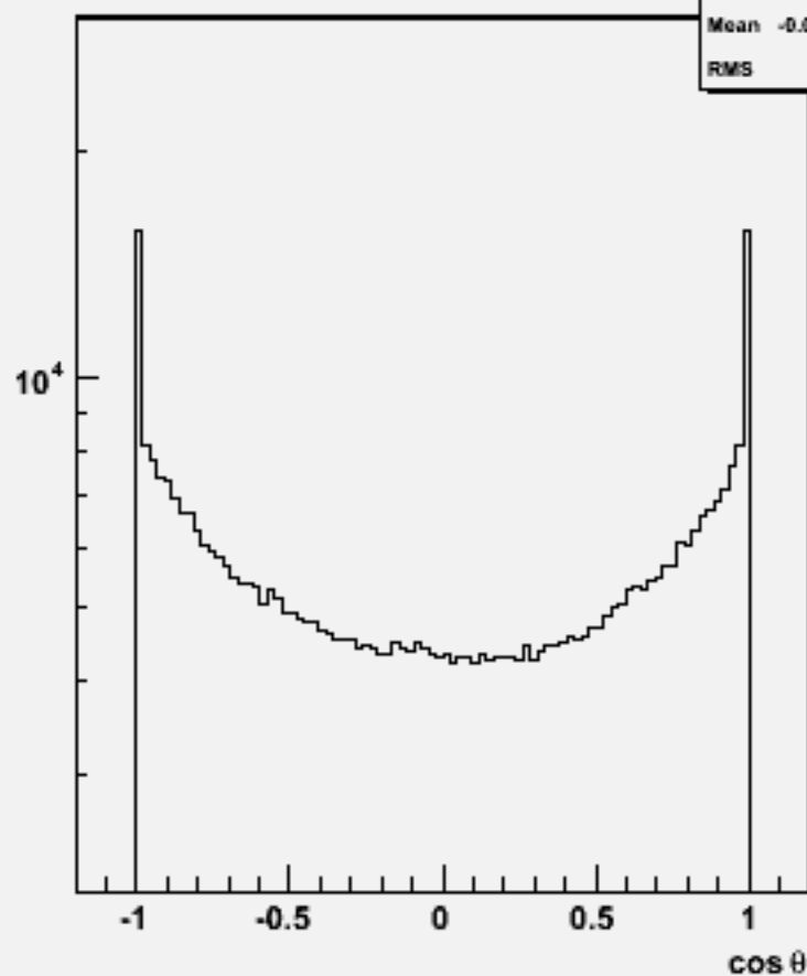
Particle cos \theta : w104000 aa_n3e3du_o
