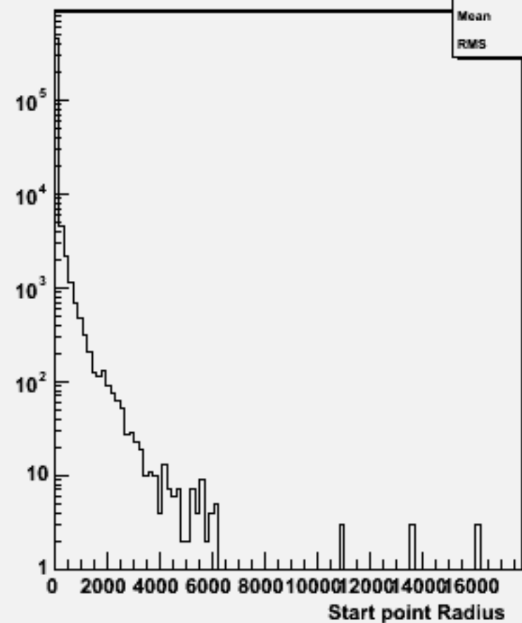
Start point R : w104000 aa_n3e3du_o
