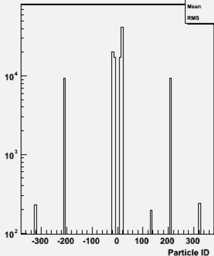
Particle ID : w103998 aa_n3e3e3n3_o
