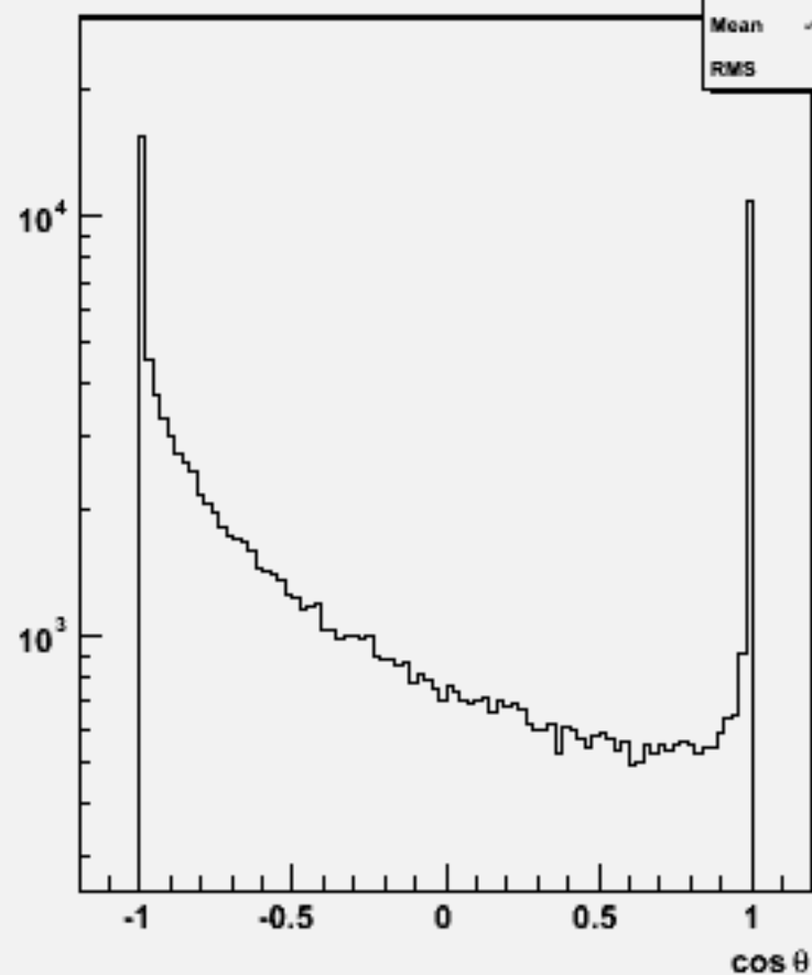
Particle cos \theta : w103998 aa_n3e3e3n3_o
