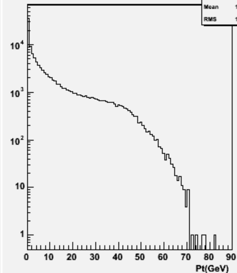
Particle Pt : w103998 aa_n3e3e3n3_o
