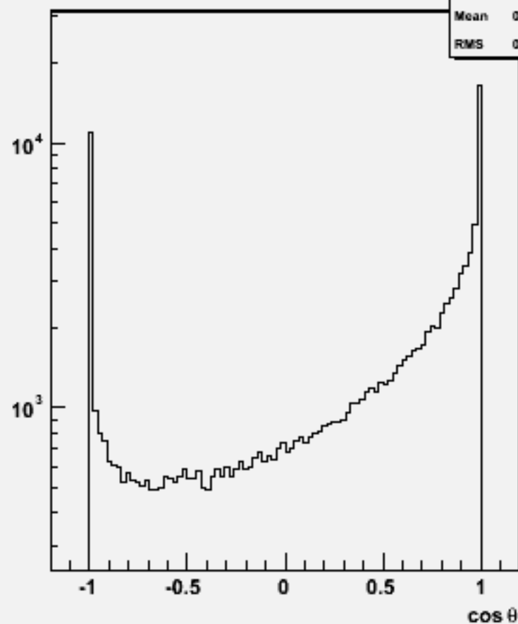
Particle cos \theta : w103997 aa_n3e3e3n3_o
