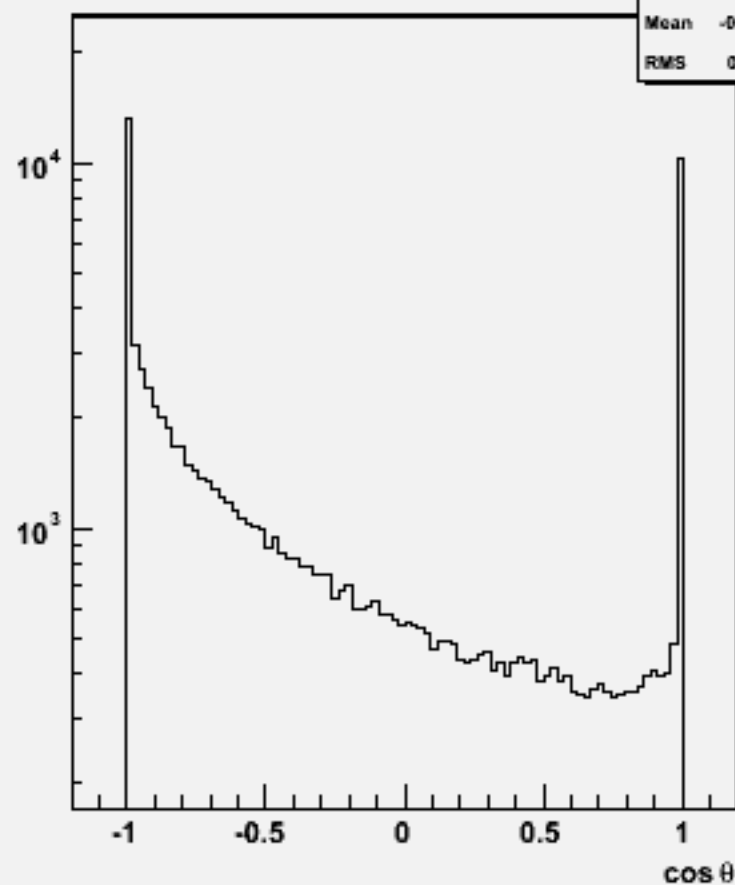
Particle cos \theta : w103994 aa_n3e3e2n2_o
