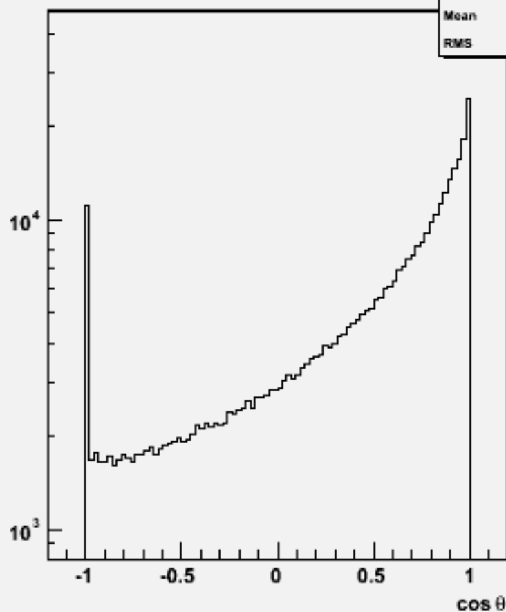
Particle cos \theta : w103981 aa_n2e2du_o
