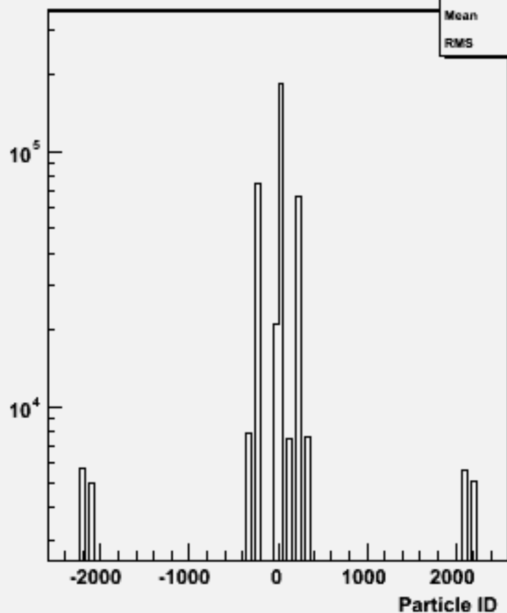
Particle ID : w103981 aa_n2e2du_o
