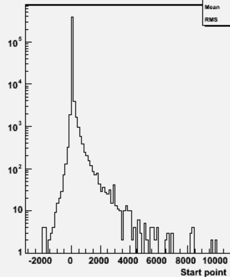
Start point Z : w103981 aa_n2e2du_o
