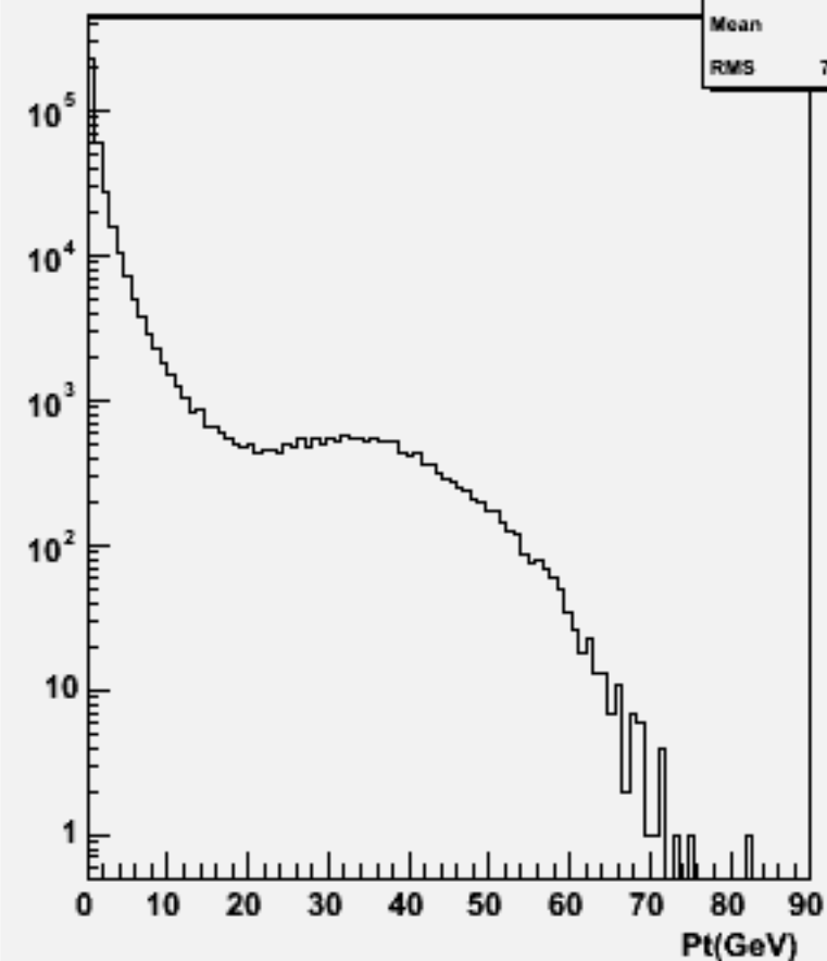
Particle Pt : w103981 aa_n2e2du_o
