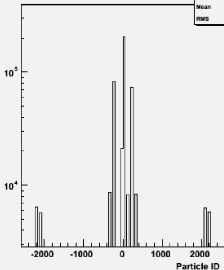
Particle ID : w103980 aa_n2e2du_o
