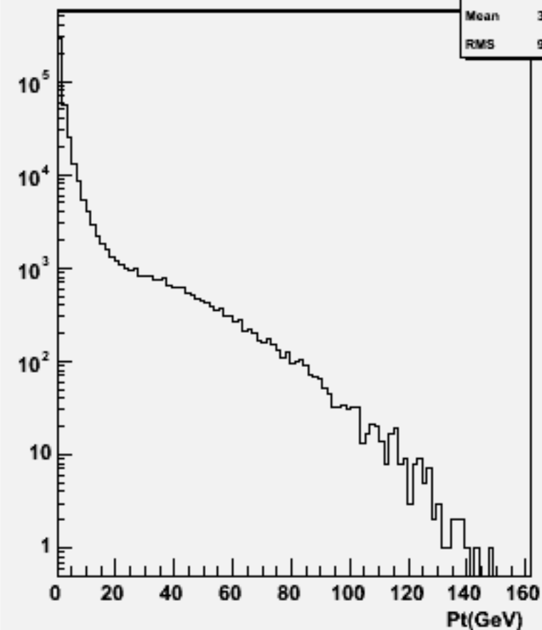
Particle Pt : w103980 aa_n2e2du_o
