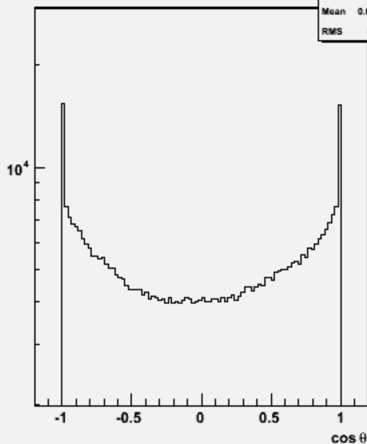
Particle cos \theta : w103980 aa_n2e2du_o
