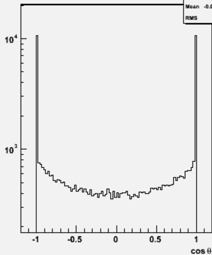
Particle cos \theta : w103972 aa_n2e2e2n2_o
