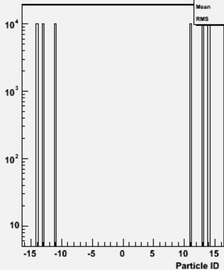
Particle ID : w103972 aa_n2e2e2n2_o
