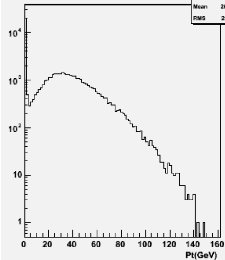
Particle Pt : w103972 aa_n2e2e2n2_o
