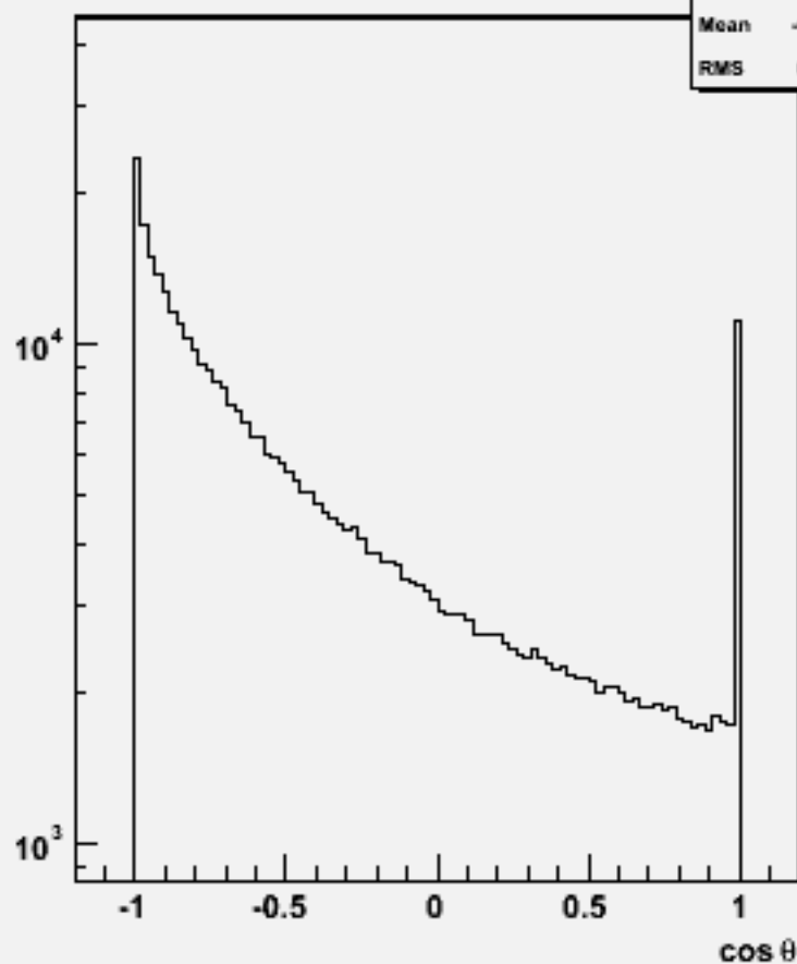
Particle cos \theta : w103962 aa_n1e1du_o
