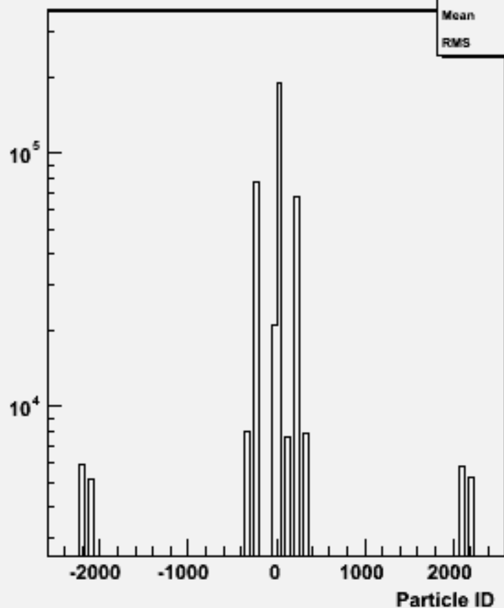
Particle ID : w103962 aa_n1e1du_o
