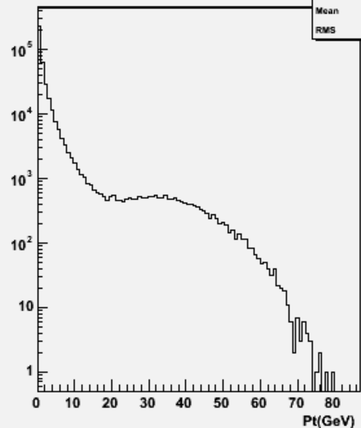
Particle Pt : w103962 aa_n1e1du_o
