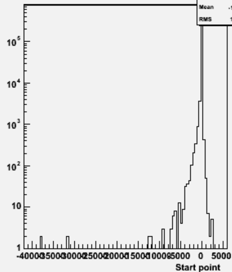
Start point Z : w103962 aa_n1e1du_o
