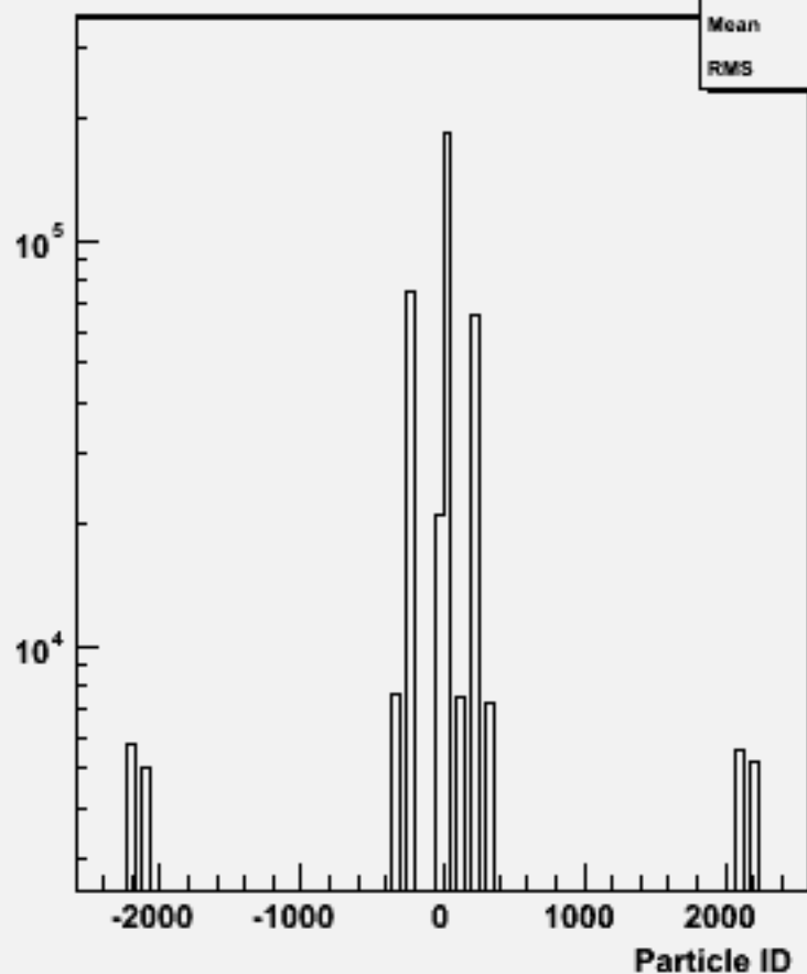
Particle ID : w103961 aa_n1e1du_o
