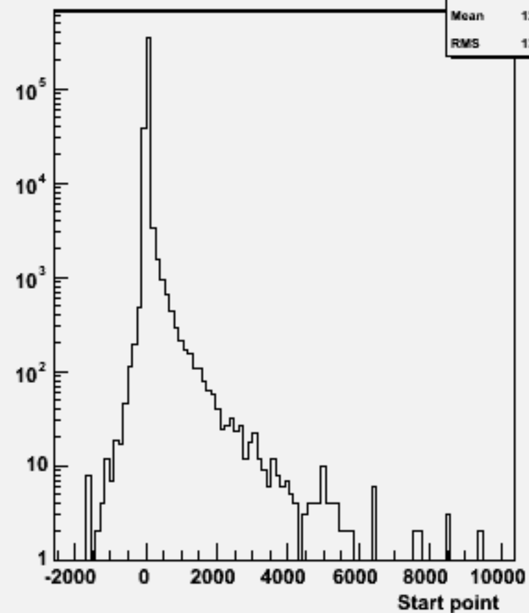
Start point Z : w103961 aa_n1e1du_o
