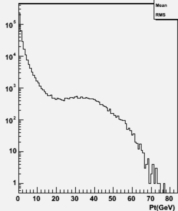
Particle Pt : w103961 aa_n1e1du_o
