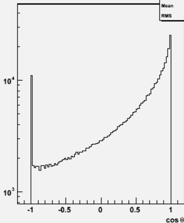
Particle cos \theta : w103961 aa_n1e1du_o
