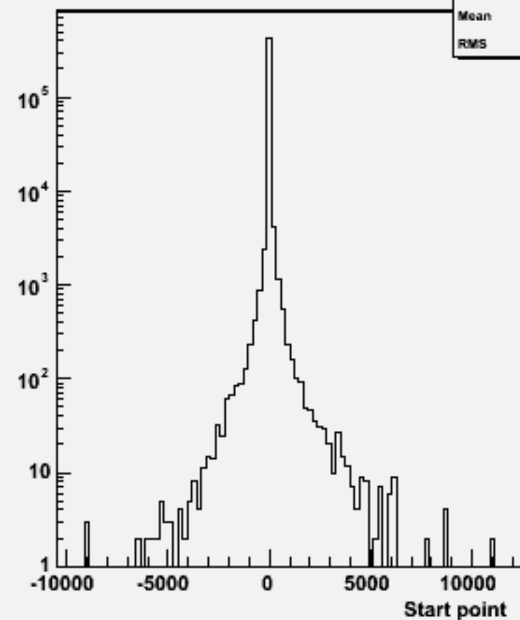
Start point Z : w103960 aa_n1e1du_o
