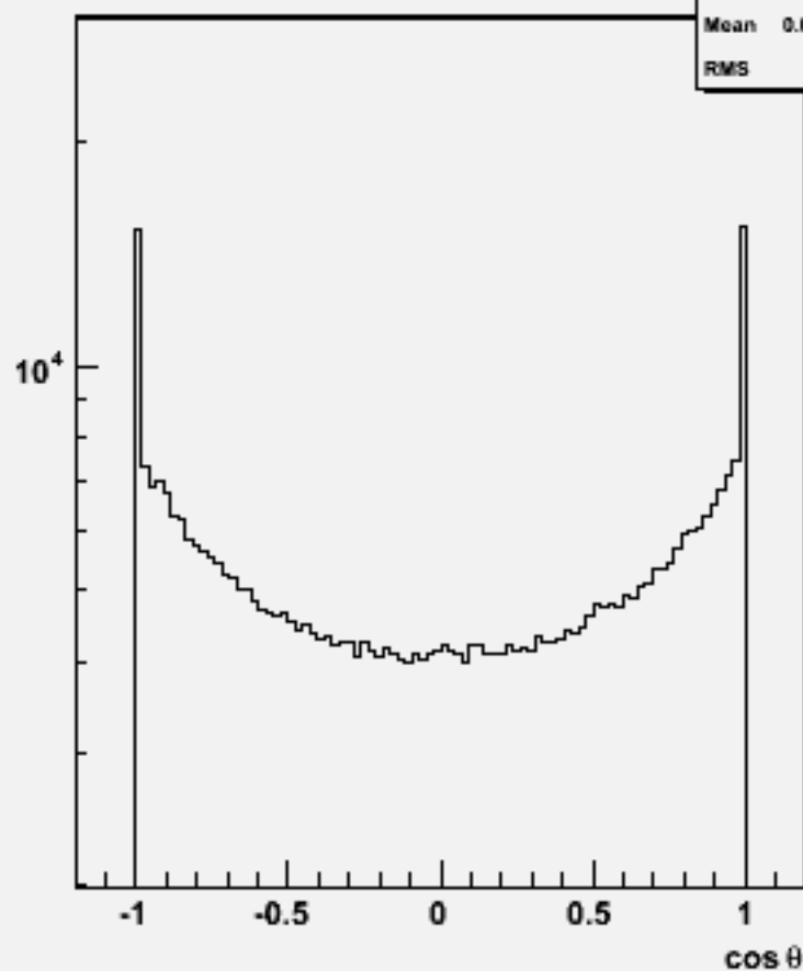
Particle cos \theta : w103960 aa_n1e1du_o
