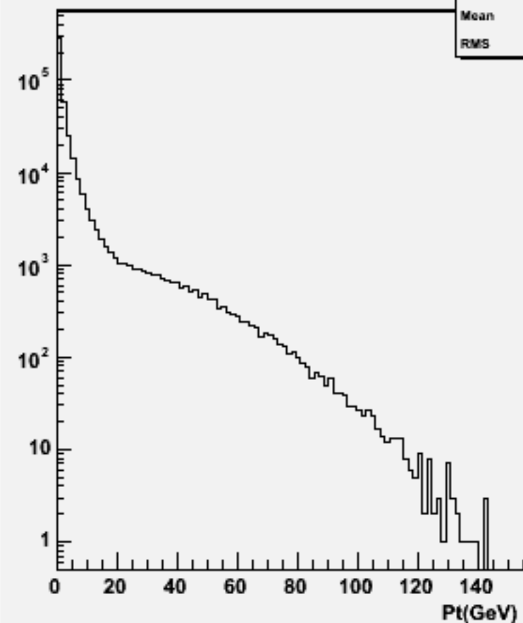
Particle Pt : w103960 aa_n1e1du_o
