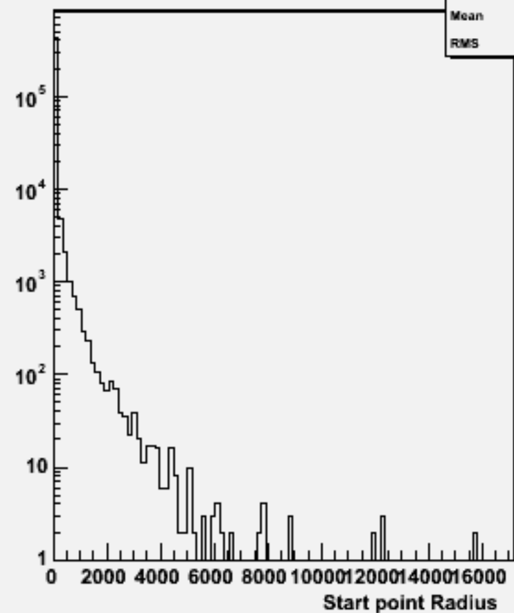
Start point R : w103960 aa_n1e1du_o
