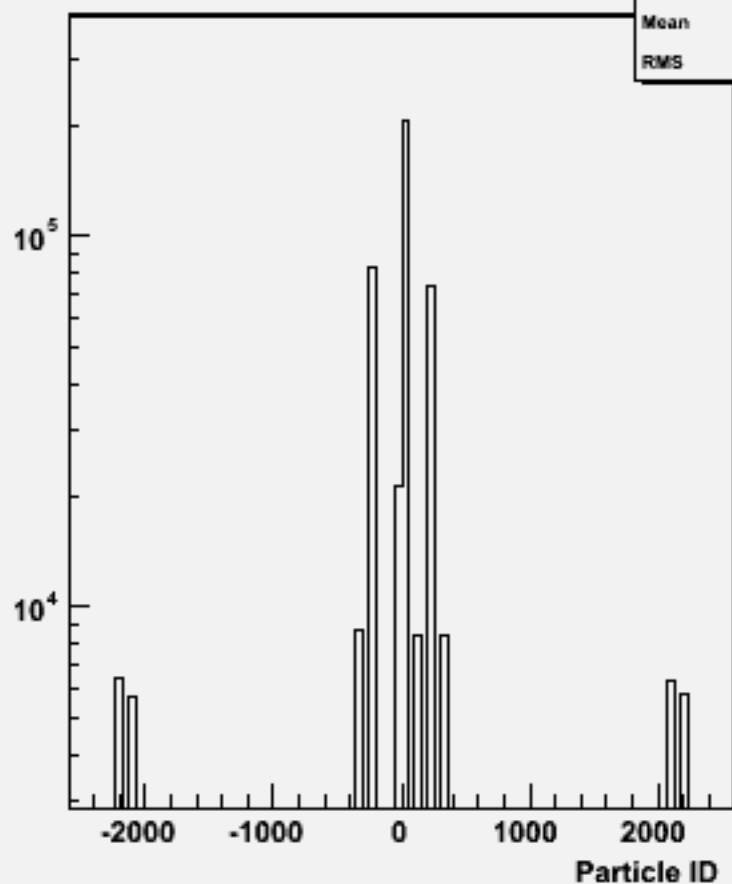
Particle ID : w103960 aa_n1e1du_o
