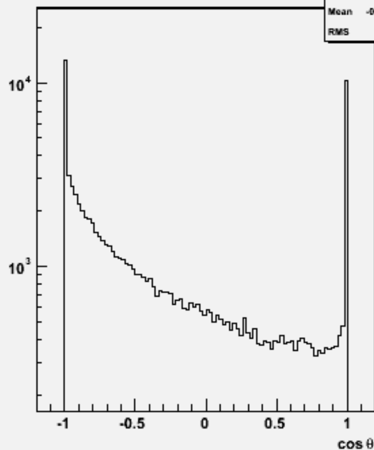
Particle cos \theta : w103958 aa_n1e1e3n3_o
