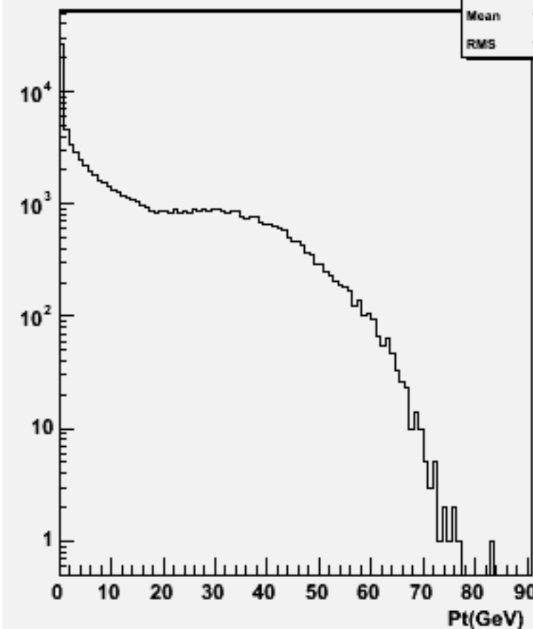
Particle Pt : w103958 aa_n1e1e3n3_o
