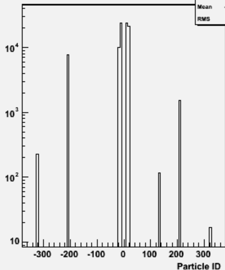
Particle ID : w103958 aa_n1e1e3n3_o
