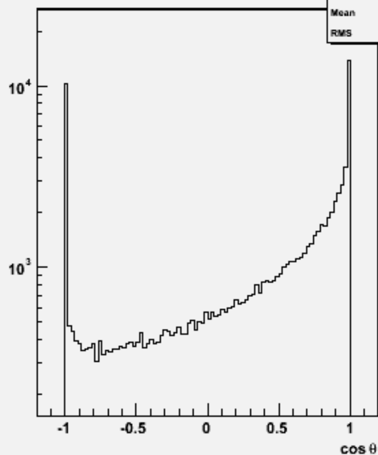
Particle cos \theta : w103957 aa_n1e1e3n3_o
