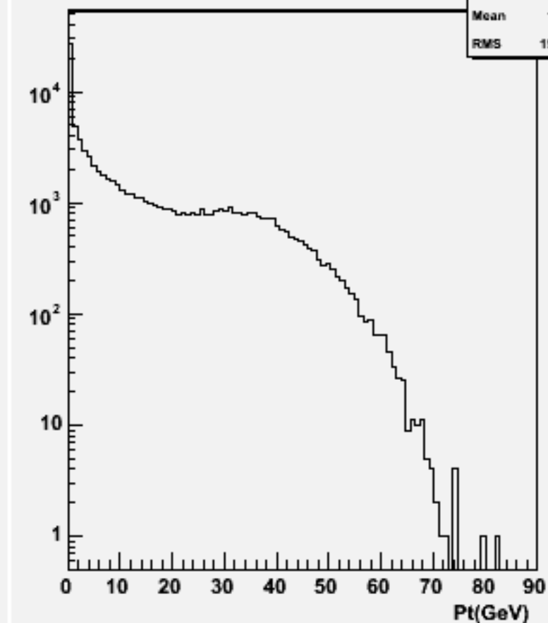
Particle Pt : w103957 aa_n1e1e3n3_o
