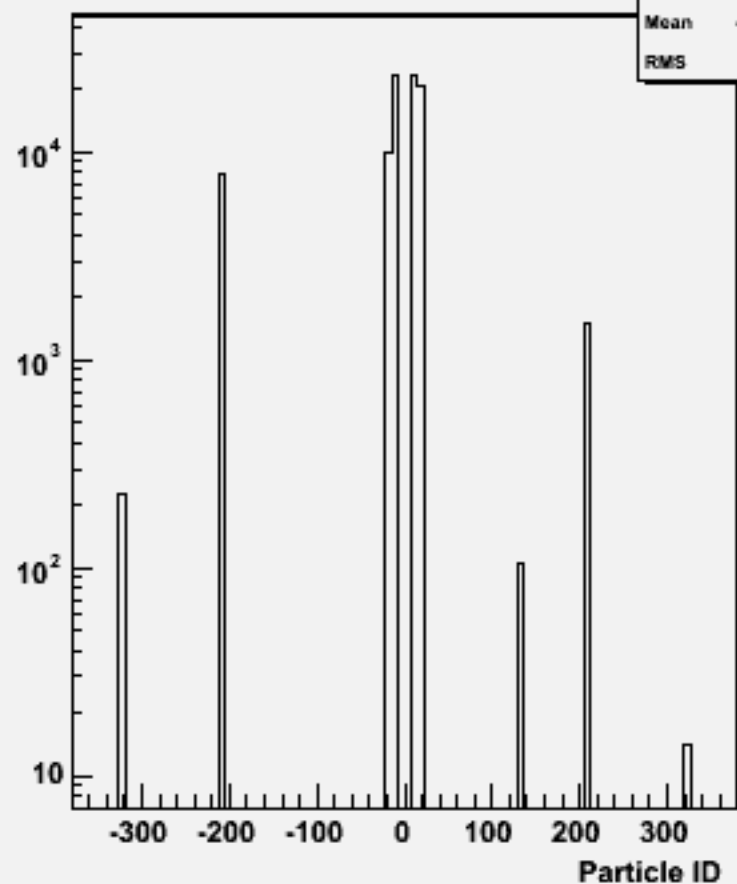
Particle ID : w103957 aa_n1e1e3n3_o
