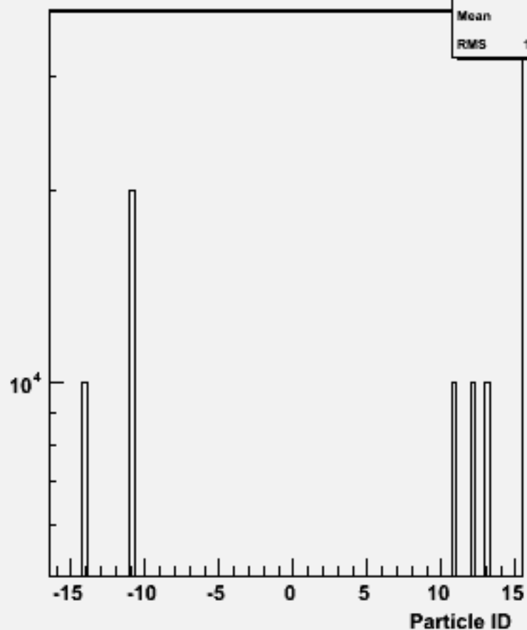
Particle ID : w103954 aa_n1e1e2n2_o
