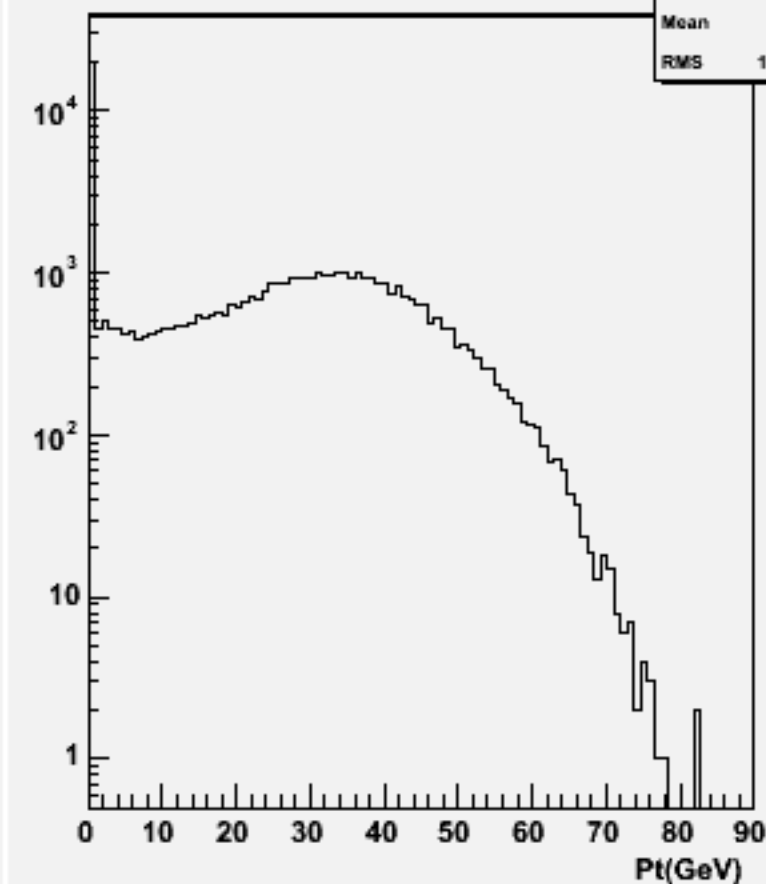
Particle Pt : w103954 aa_n1e1e2n2_o
