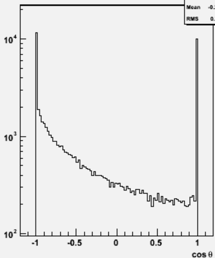
Particle cos \theta : w103954 aa_n1e1e2n2_o
