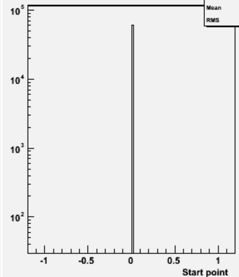
Start point Z : w103954 aa_n1e1e2n2_o
