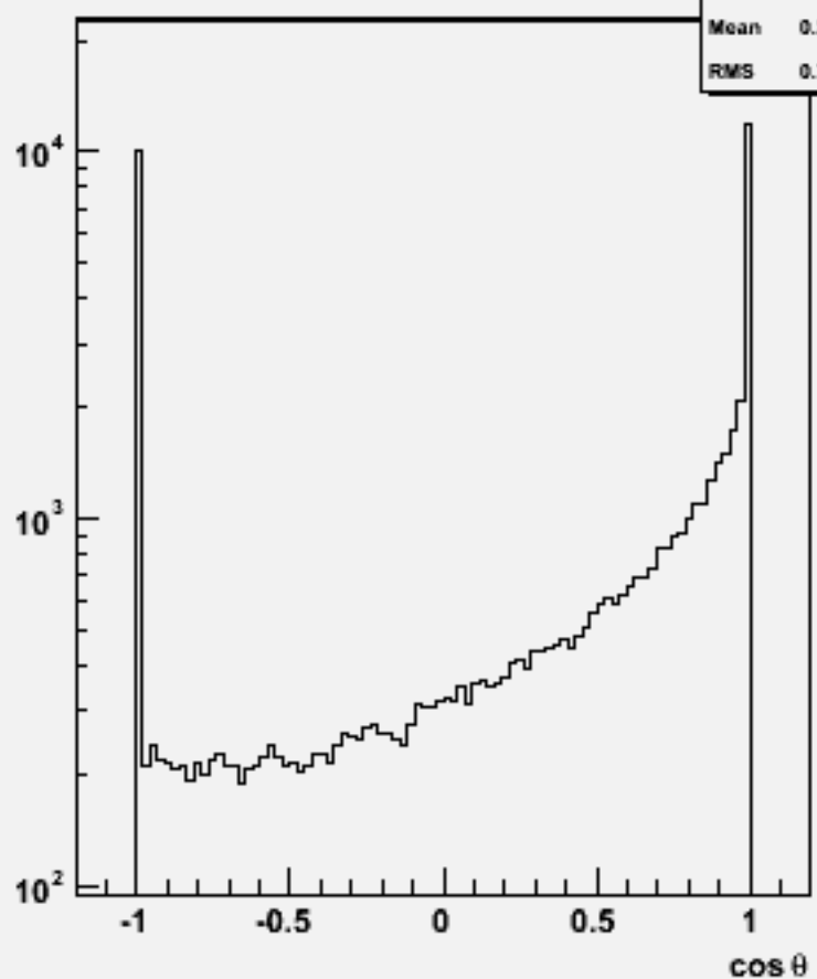
Particle cos \theta : w103953 aa_n1e1e2n2_o
