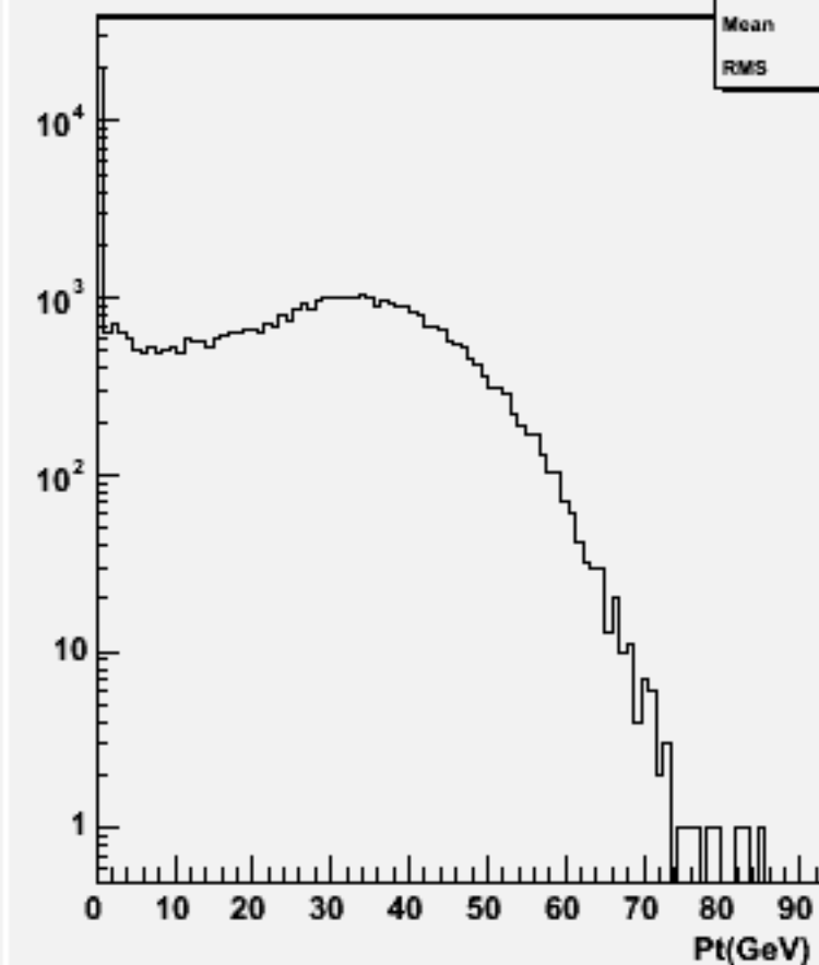
Particle Pt : w103953 aa_n1e1e2n2_o
