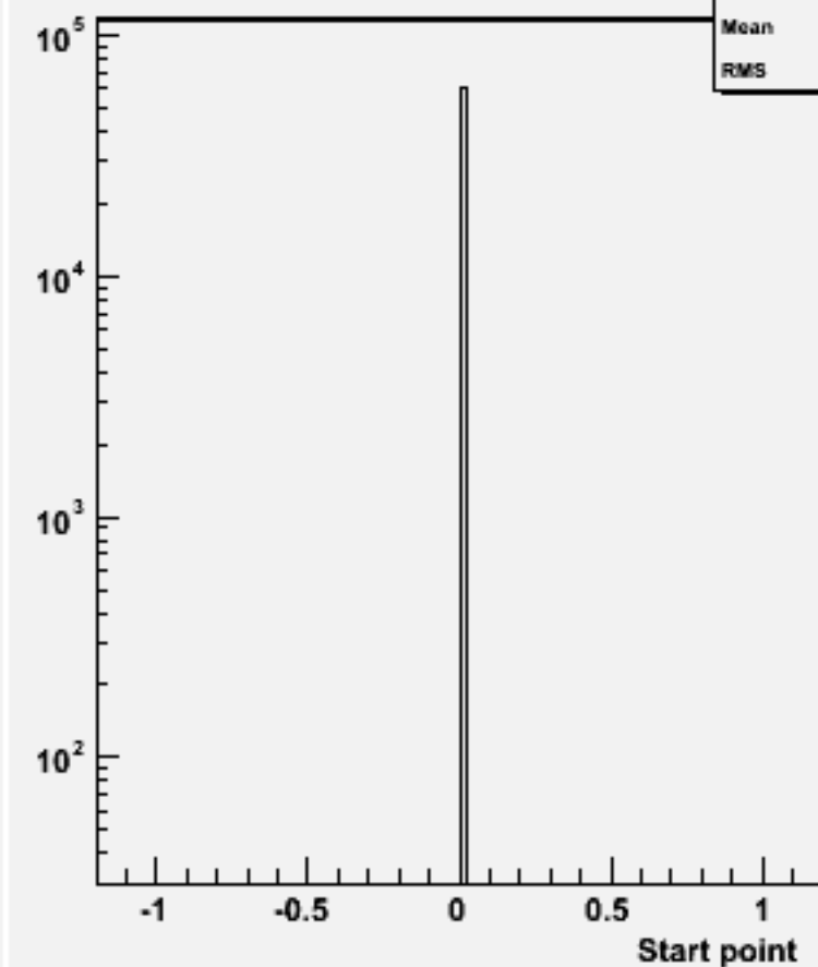
Start point Z : w103953 aa_n1e1e2n2_o
