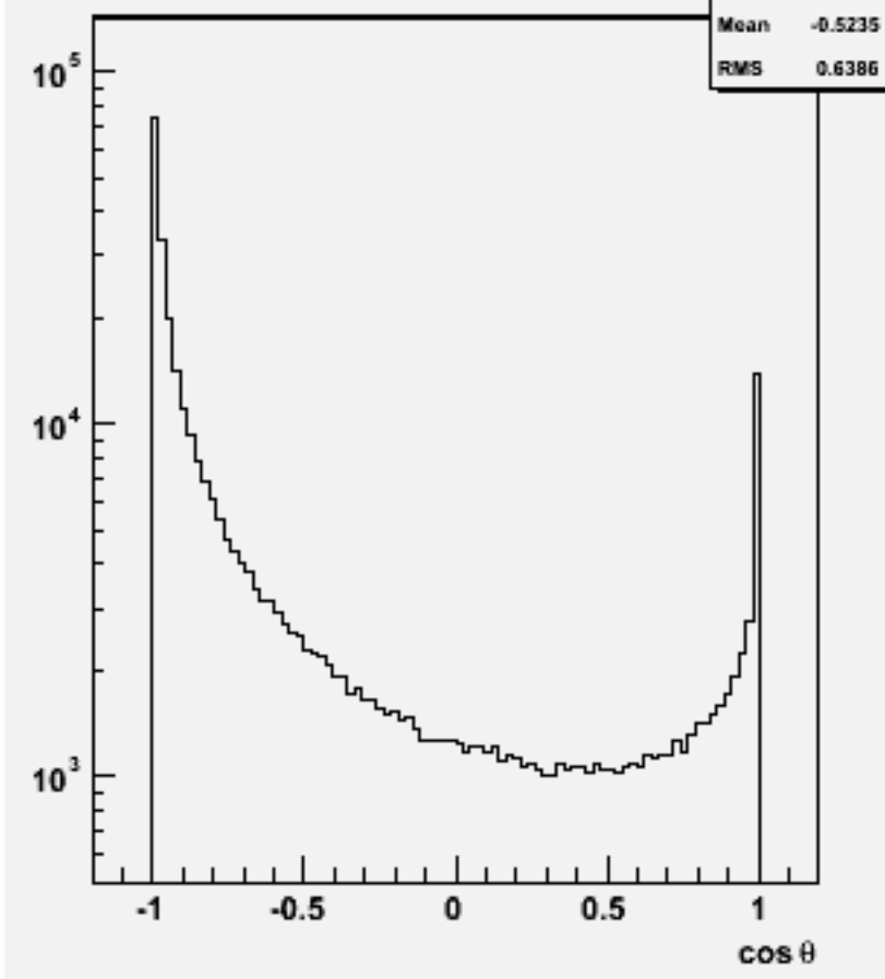
Particle cos \theta : w103919 ae1_e1e3e3ss_o
