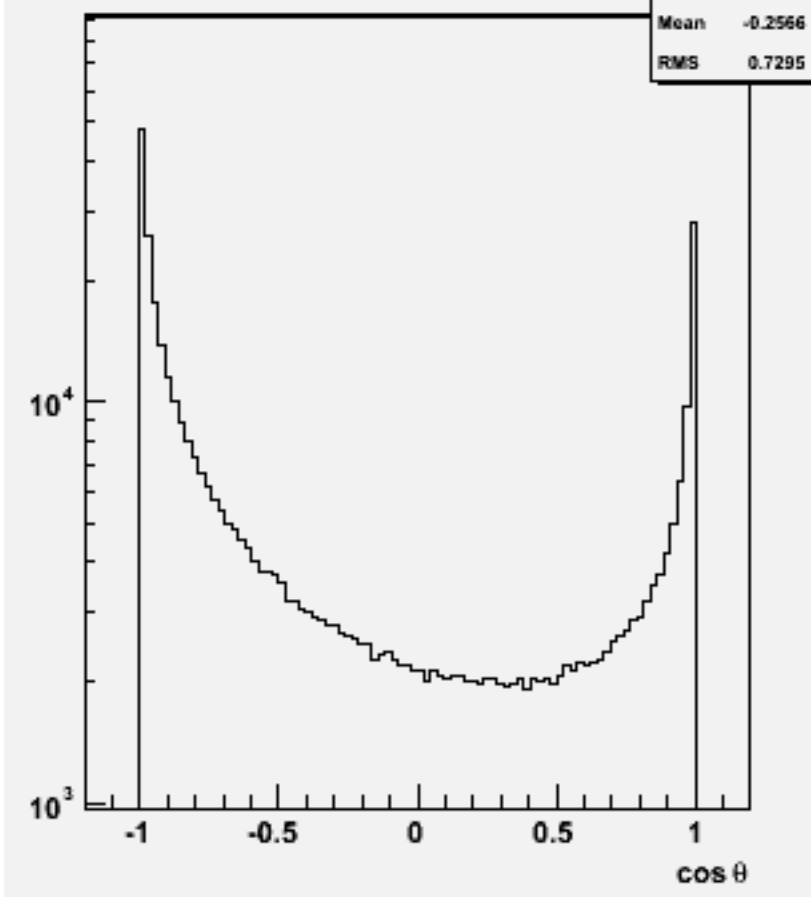
Particle cos \theta : w103918 ae1_e1e3e3ss_o
