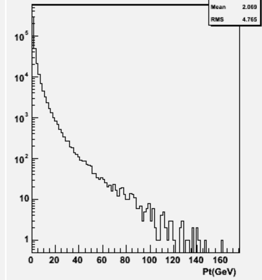
Start point Z : w103918 ae1_e1e3e3ss_o
