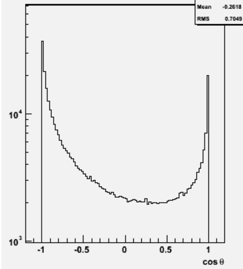
Particle cos θ : w103902 ae1_e1e2e2ss_o
