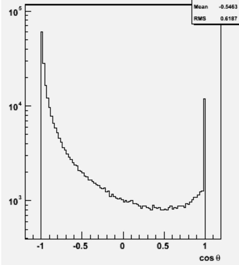
Particle cos θ : w103901 ae1_e1e2e2ss_o
