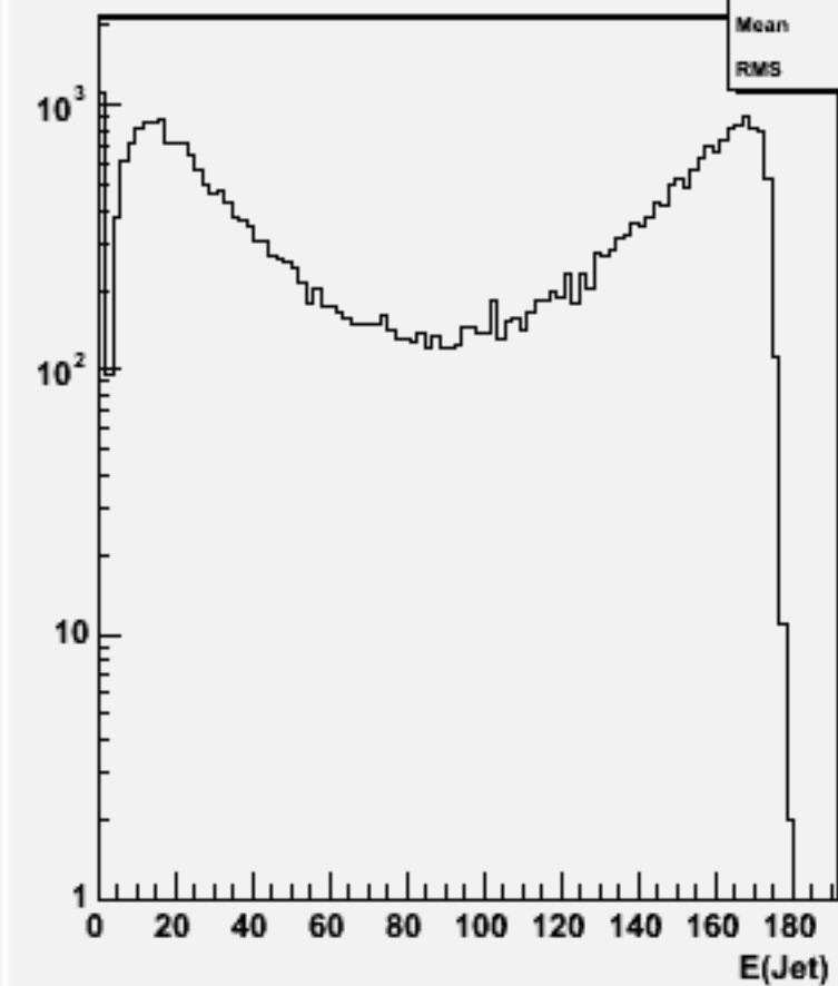
Jet energies(All jets)w103888 ae1_e1e2e2e2_o
