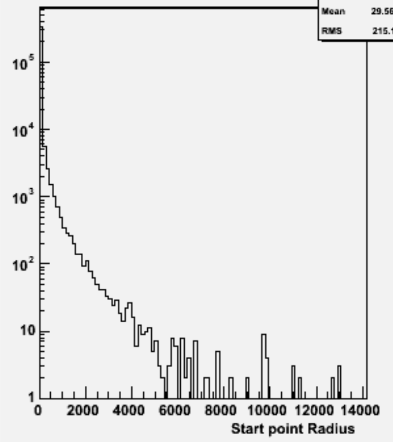
Start point R : w103880 ae1_e1e1e1ss_o
