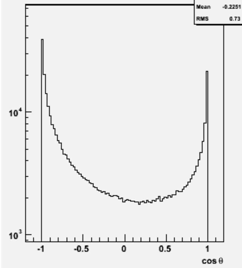
Particle cos \theta : w103880 ae1_e1e1e1ss_o
