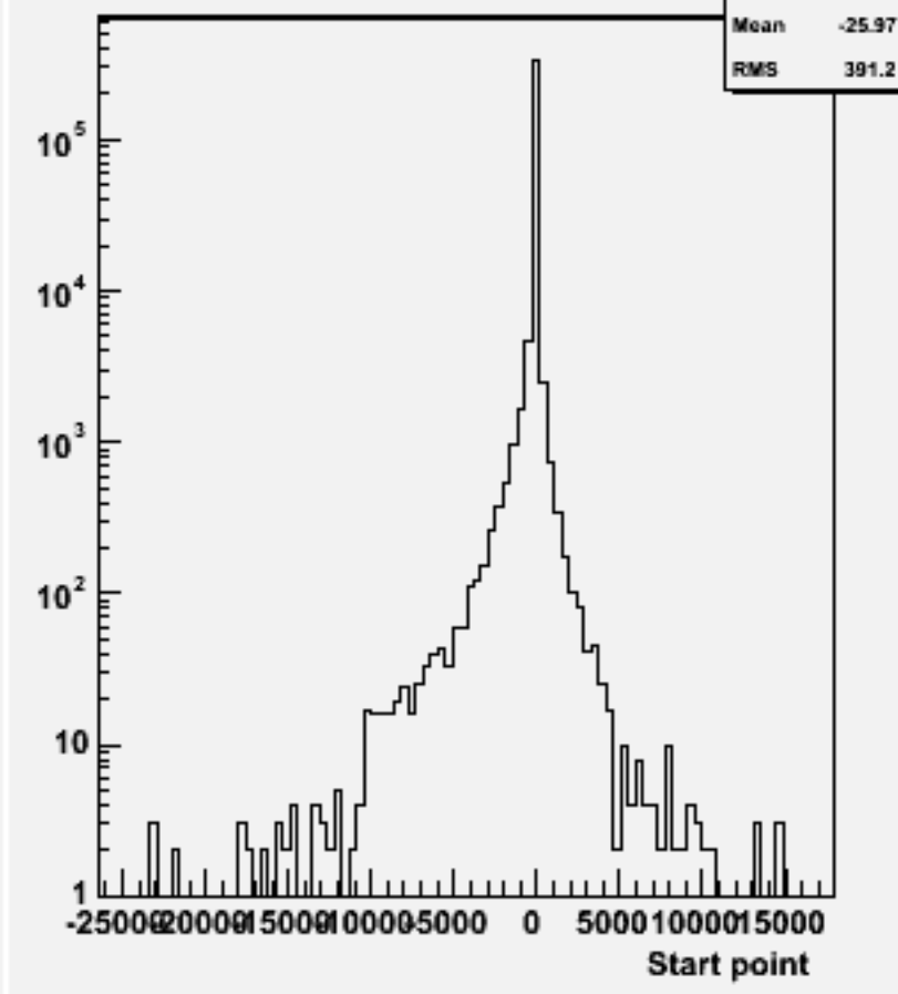
Start point Z : w103880 ae1_e1e1e1ss_o
