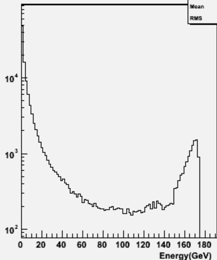
Start point R : w103873 ae1_e1e1e1e3e3_o
