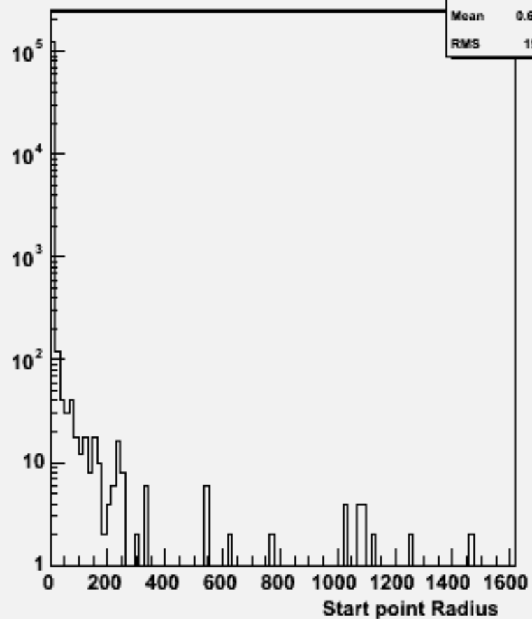
Start point R : w103873 ae1_e1e1e1e3e3_o
