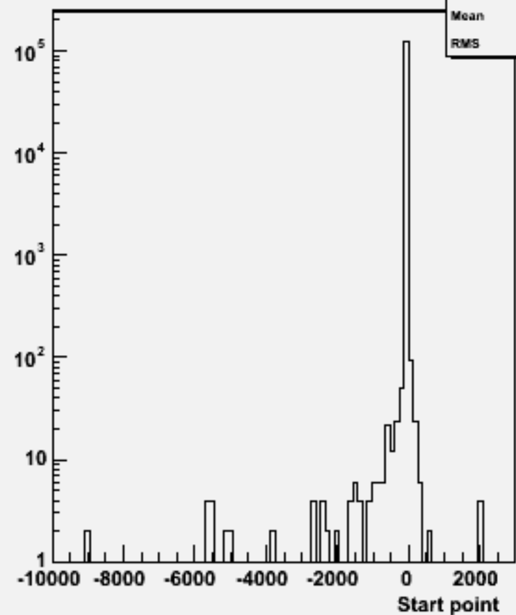
Start point Z : w103873 ae1_e1e1e1e3e3_o
