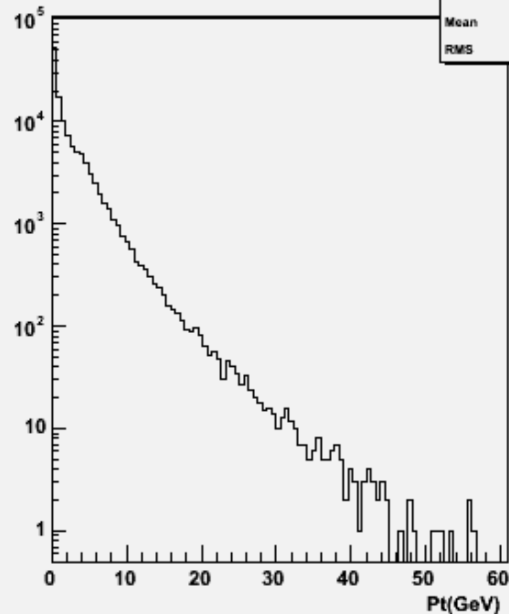
Particle Pt : w103873 ae1_e1e1e1e3e3_o
