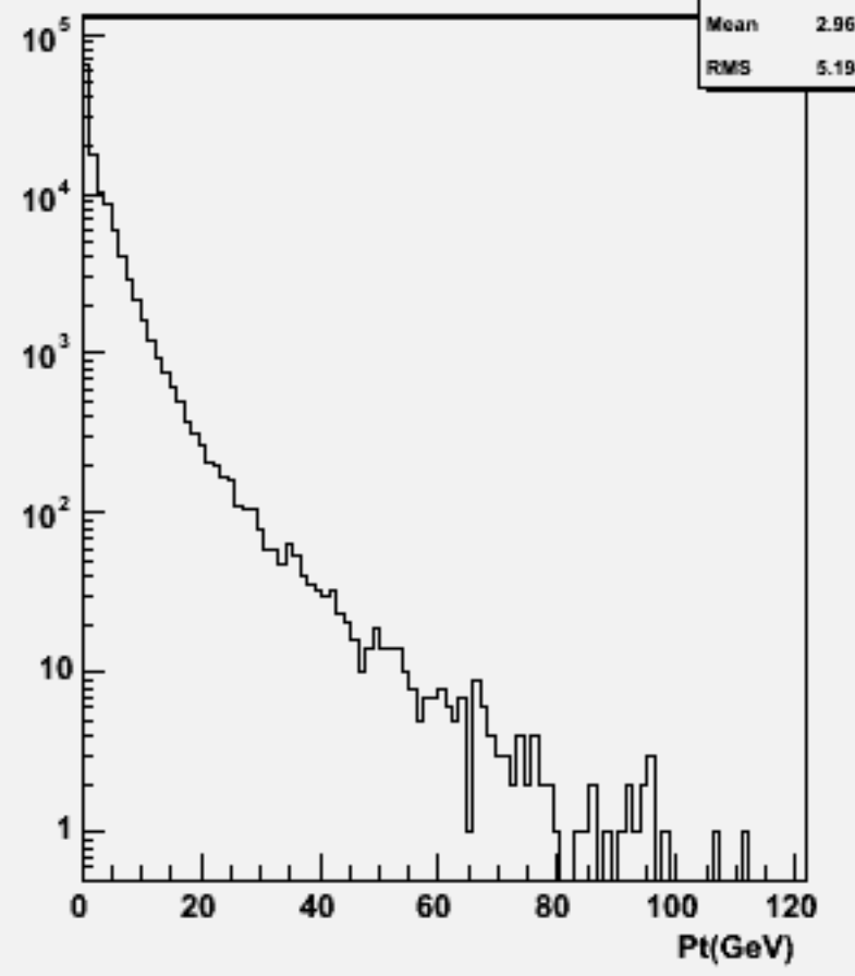
Start point Z : w103872 ae1_e1e1e1e3e3_o
