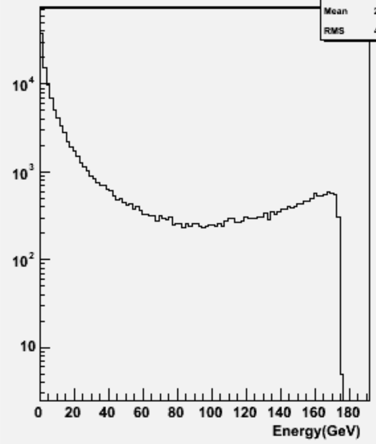
Start point R : w103872 ae1_e1e1e1e3e3_o
