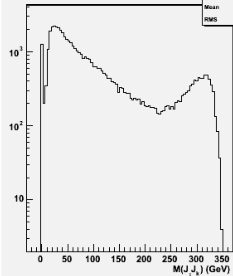
2jets mass(All comb)w103870 ae1_e1e1e1e2e2_o
