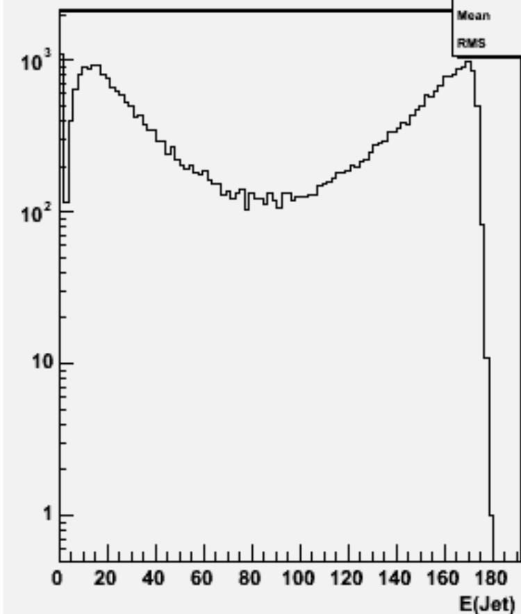
Jet energies(All jets)w103870 ae1_e1e1e1e2e2_o
