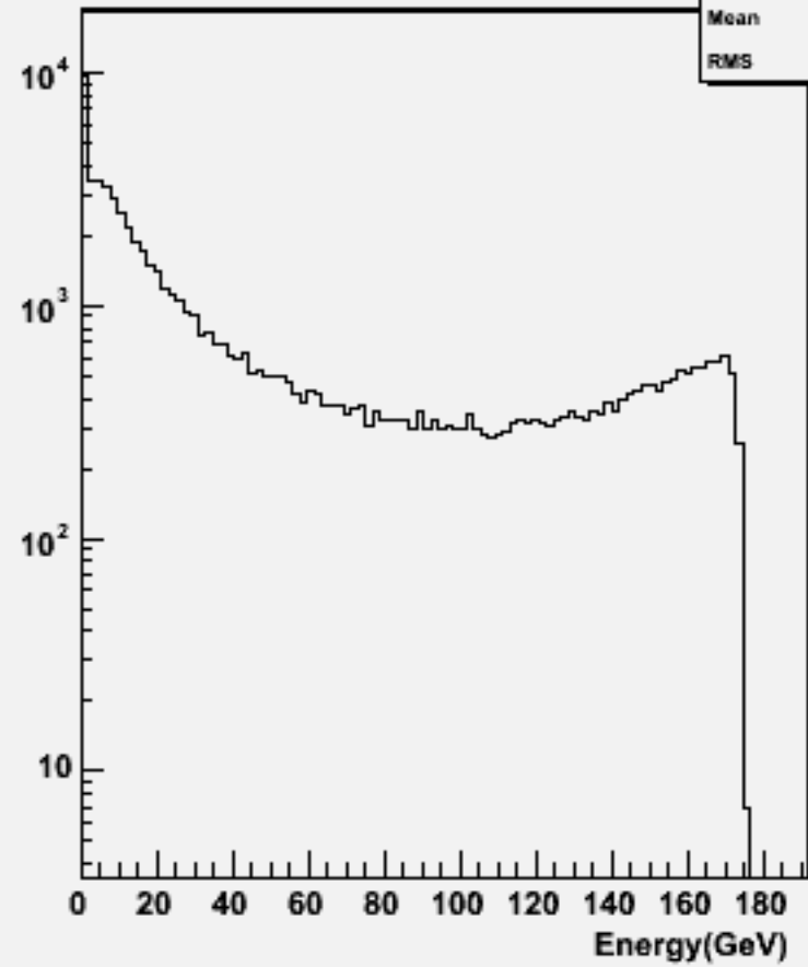
Particle Energy : w103868 ae1_e1e1e1e2e2_o
