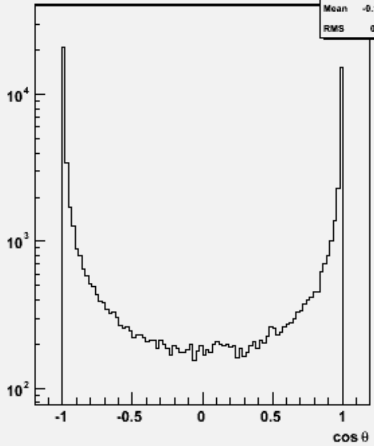
Particle cos \theta : w103868 ae1_e1e1e1e2e2_o
