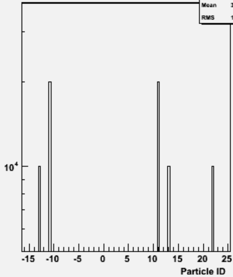
Particle ID : w103868 ae1_e1e1e1e2e2_o
