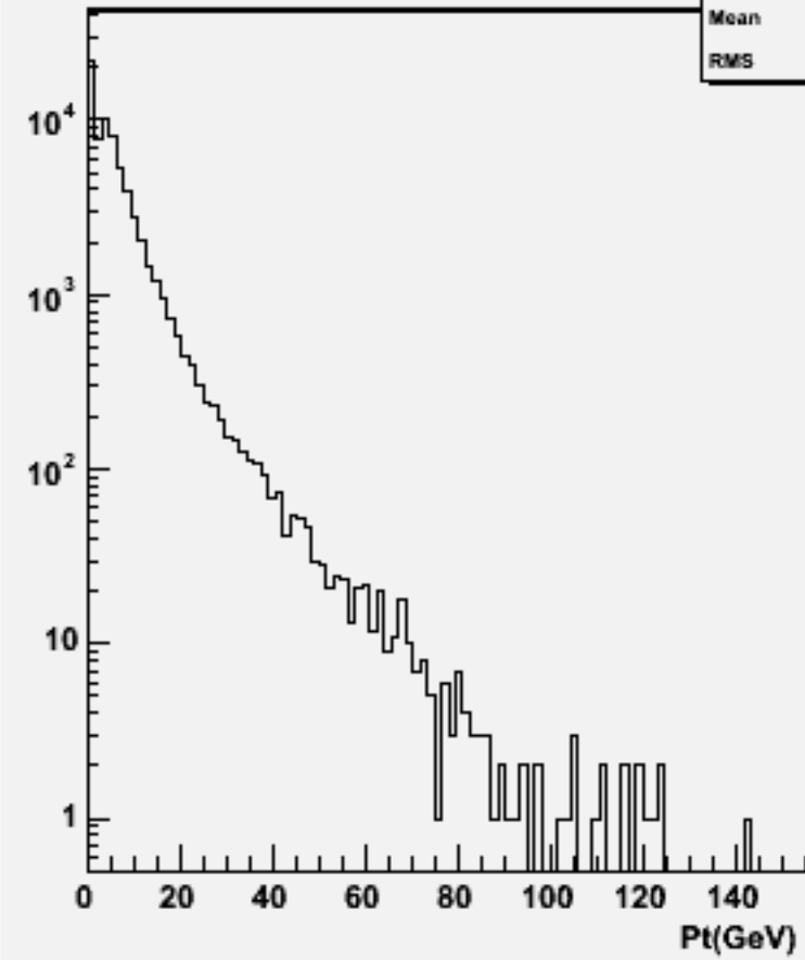
Particle Pt : w103868 ae1_e1e1e1e2e2_o
