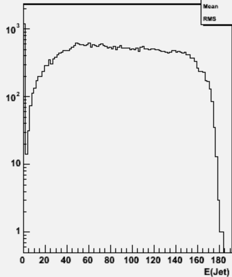
Jet energies(All jets)w103838 ae1_e1uuss_o
