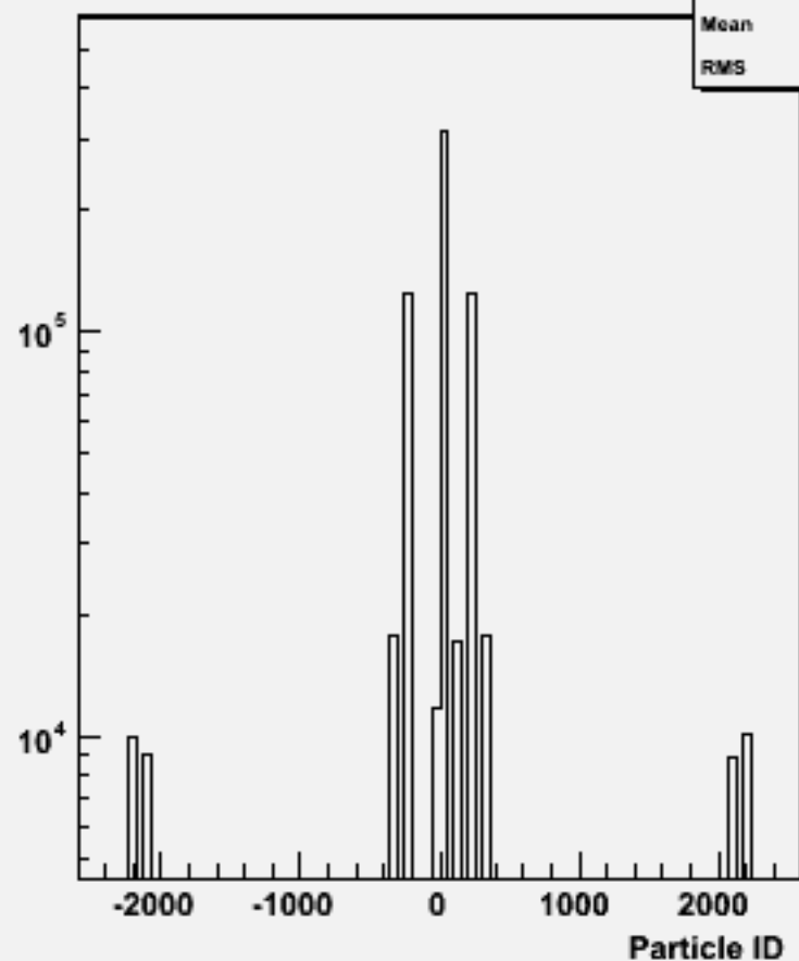
Particle ID : w103836 ae1_e1uuss_o
