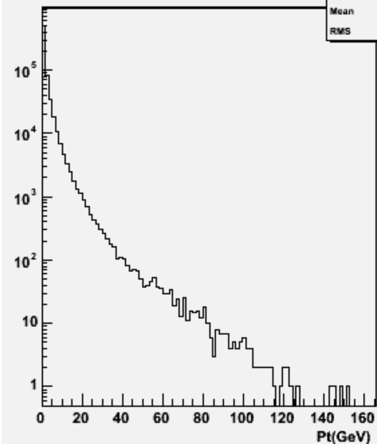
Particle Pt : w103836 ae1_e1uuss_o
