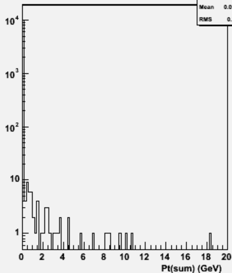
Pt Sum: w103836 ae1_e1uuss_o
