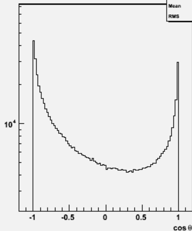
Particle cosθ : w103836 ae1_e1uuss_o
