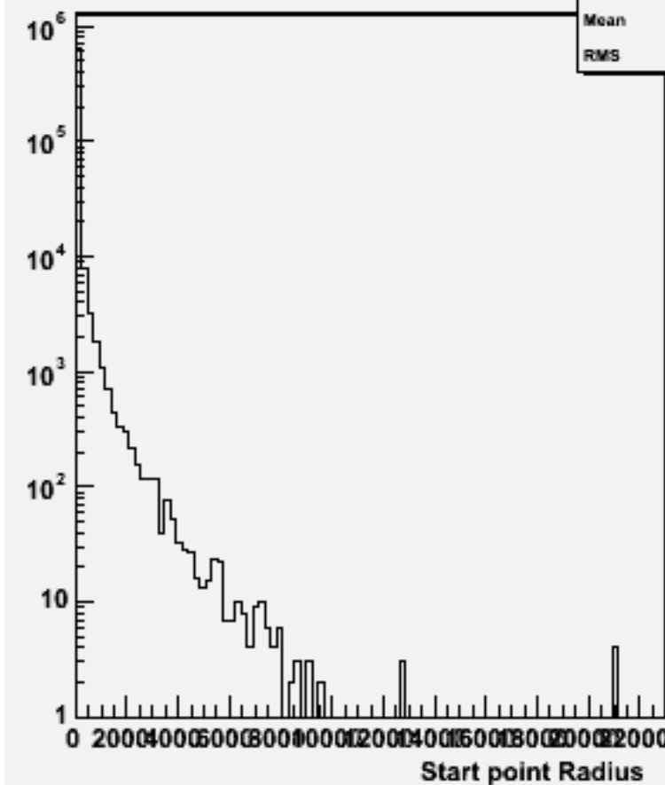
Start point R : w103836 ae1_e1uuss_o
