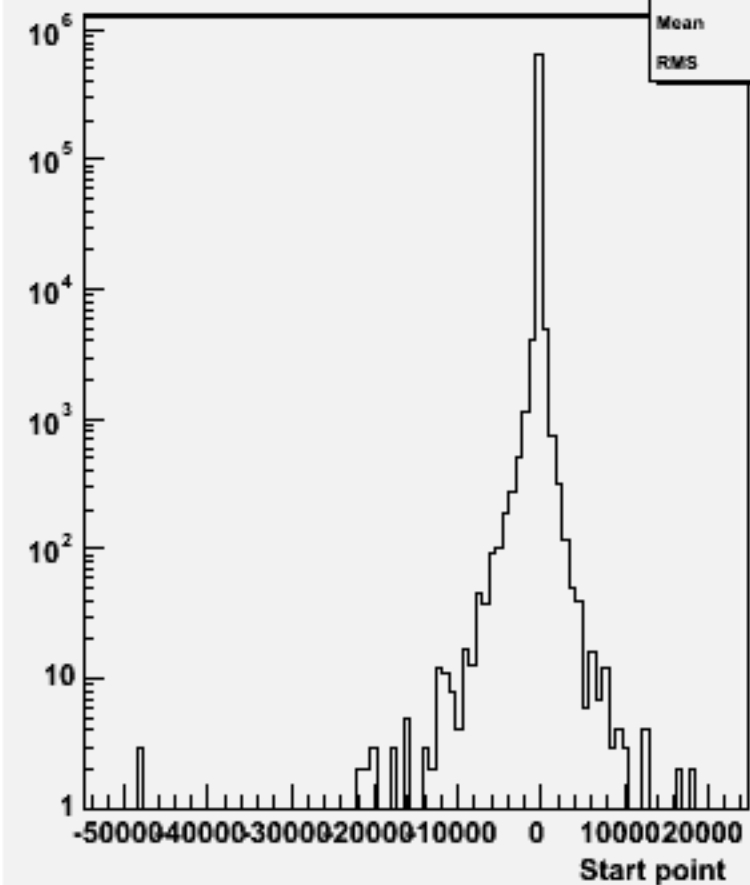
Start point Z : w103836 ae1_e1uuss_o
