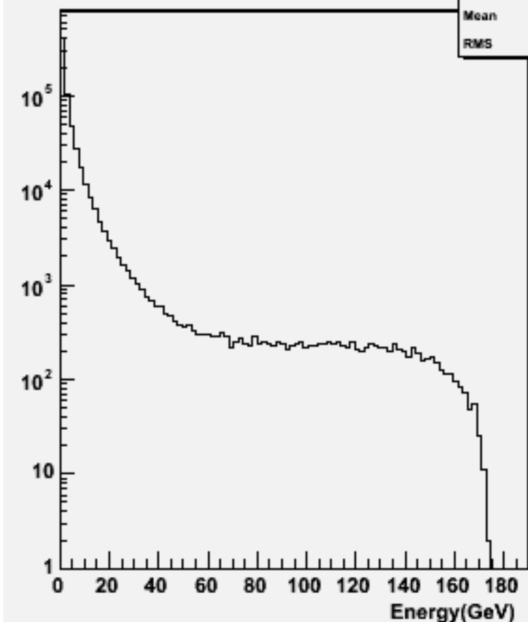
Particle Energy : w103836 ae1_e1uuss_o
