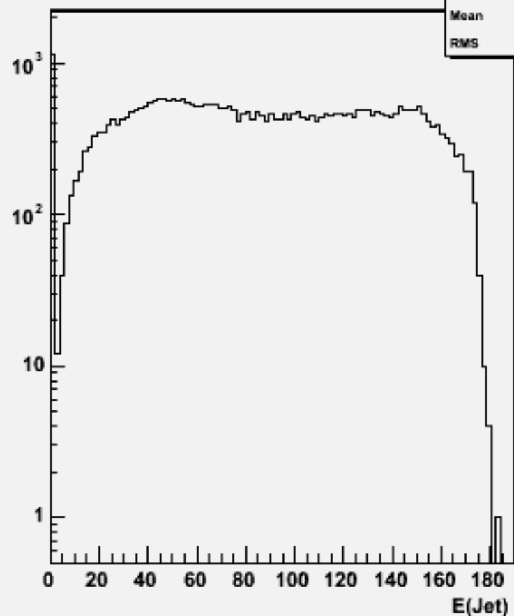
Jet energies(All jets)w103836 ae1_e1uuss_o
