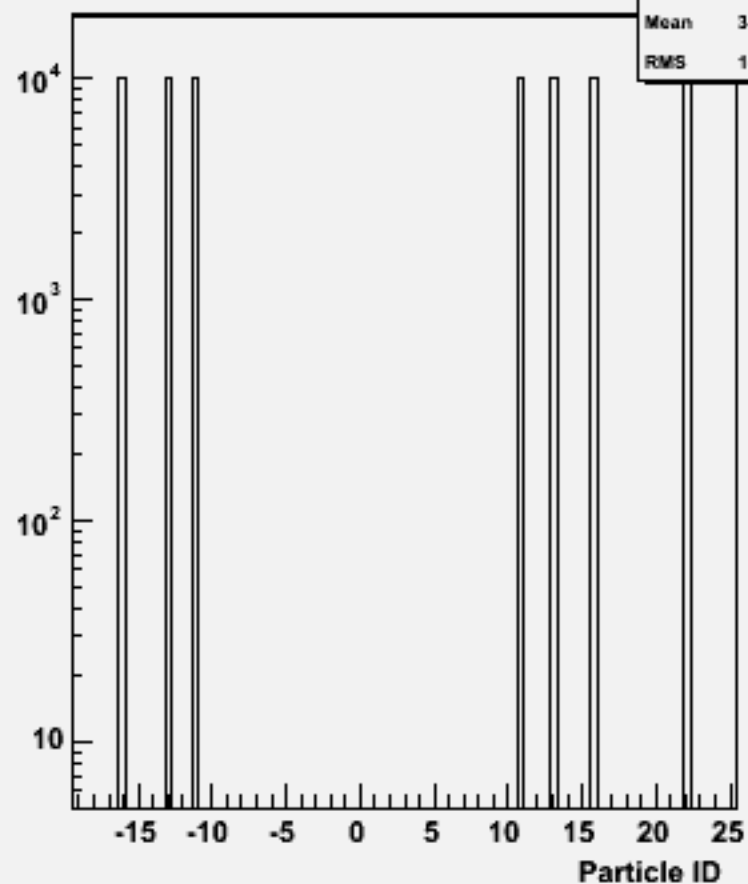
Particle ID : w103808 ae1_e1n3n3e2e2_o
