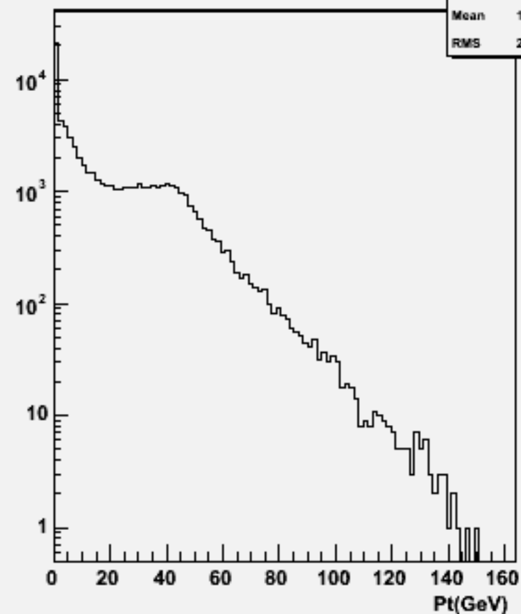
Particle Pt : w103808 ae1_e1n3n3e2e2_o
