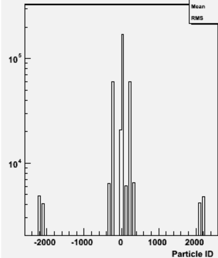
Particle ID : w103764 ae1_e1n3n3uu_o
