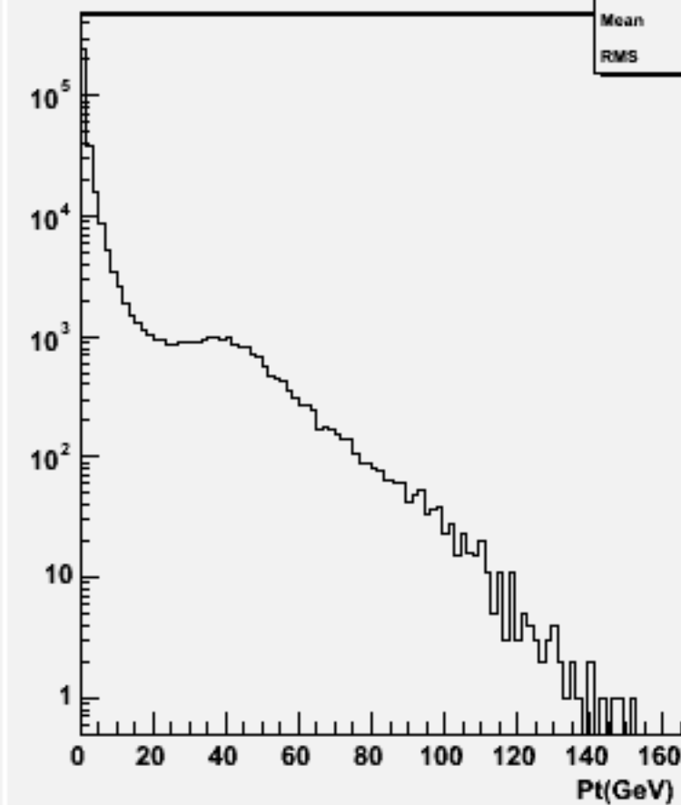
Particle Pt : w103764 ae1_e1n3n3uu_o
