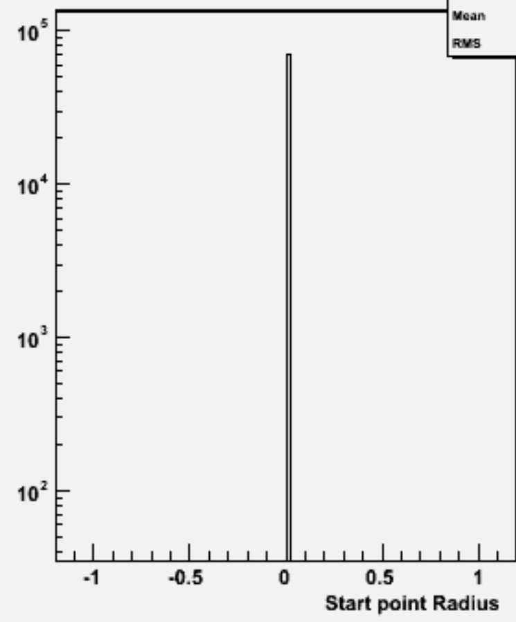
Start point R : w103669 ae1_e1n2e2e2n2_o
