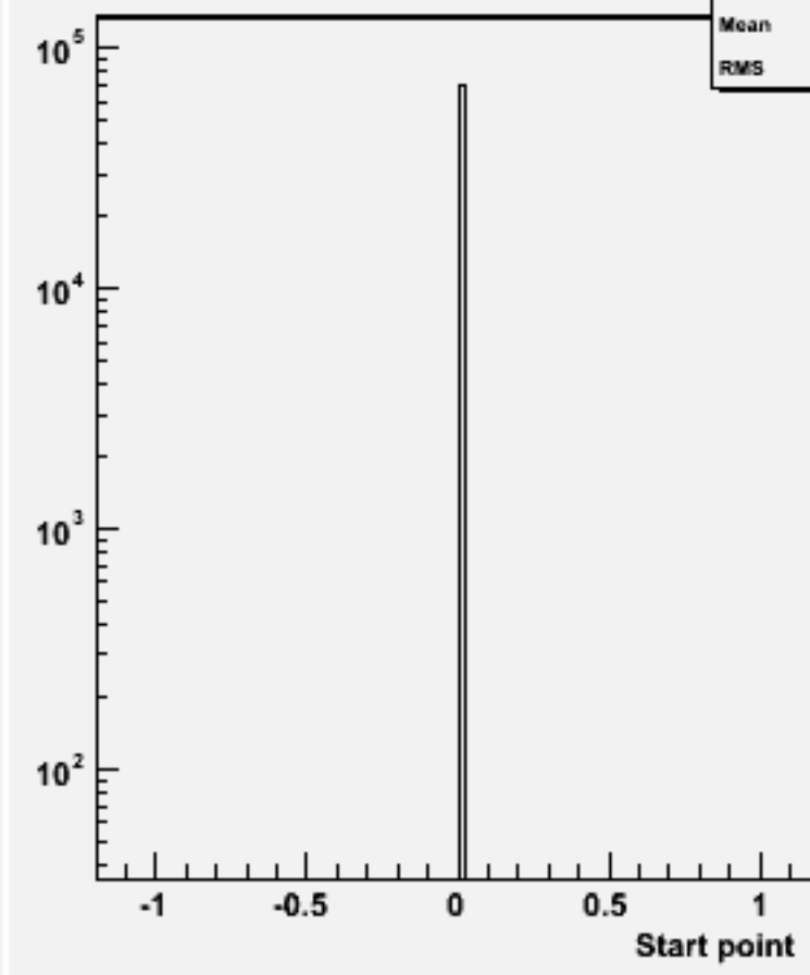
Start point Z : w103669 ae1_e1n2e2e2n2_o
